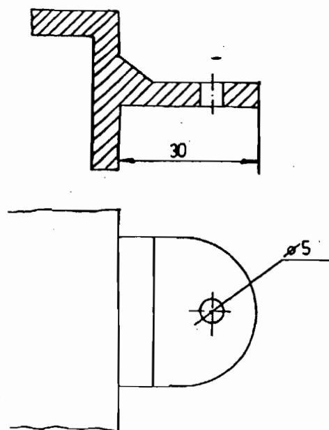
DETALLE D
