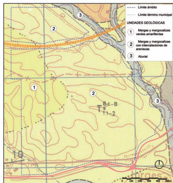
UNIDADES GEOLÓGICAS
