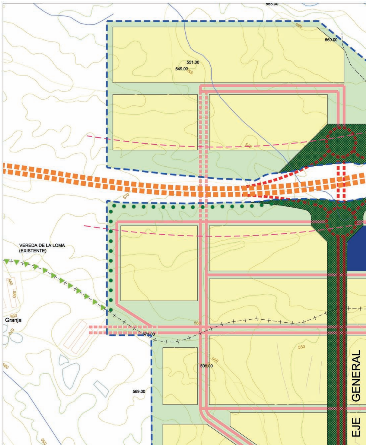
PROYECTO DE ACTUACIÓN PARA LA DECLARACIÓN DE INTERÉS AUTONÓMICO DEL "PARQUE DE INNOVACIÓN EMPRESARIAL DEL MÁRMOL". PURCHENA-URRÁCAL (ALMERÍA). Plano de Ordenación 0.3. SISTEMAS GENERALES Y ESTRUCTURA ORGÁNICA. Hoja 1
