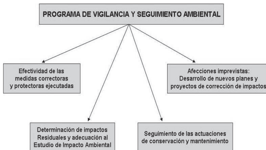
FIGURA 26: ESQUEMA METODOLÓGICO DE LA TERCERA FASE DEL PROGRAMA DE SEGUIMIENTO Y VIGILANCIA AMBIENTAL
