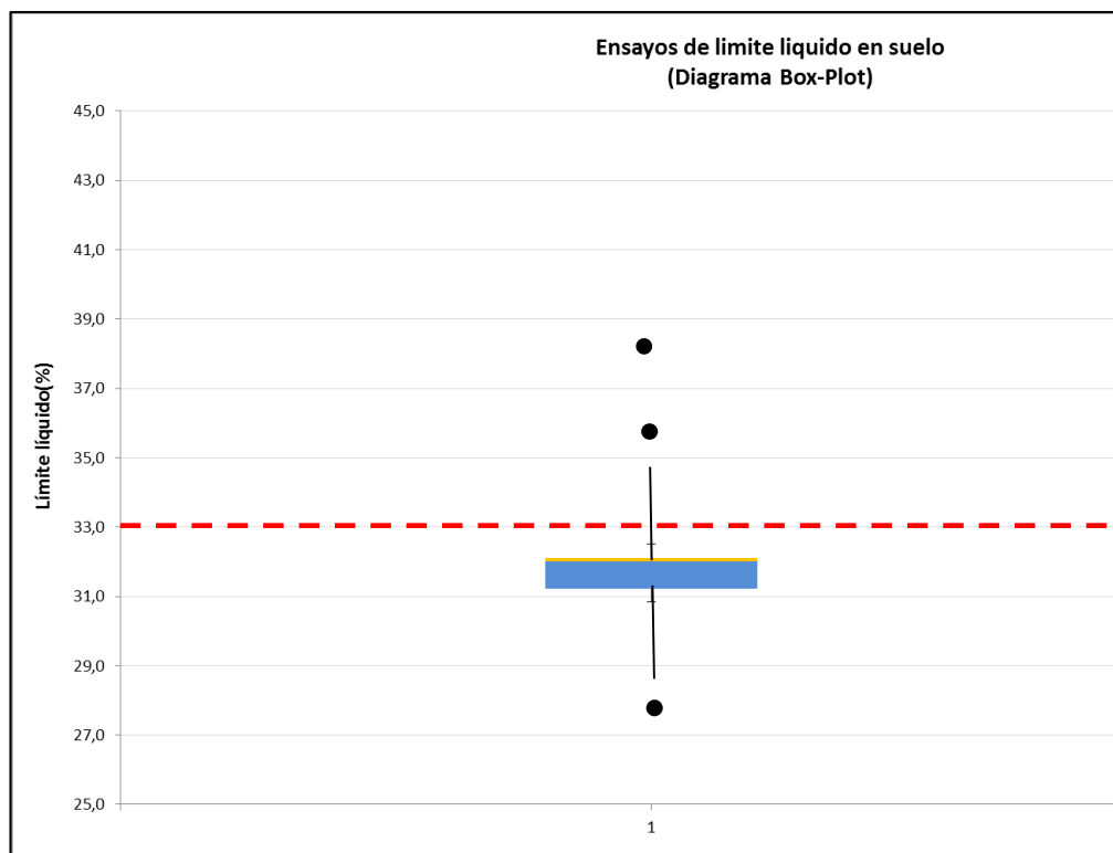
Gráfico 12. Diagrama de cajas y bigotes del ensayo del límite líquido en suelo a nivel comunidad autónoma
