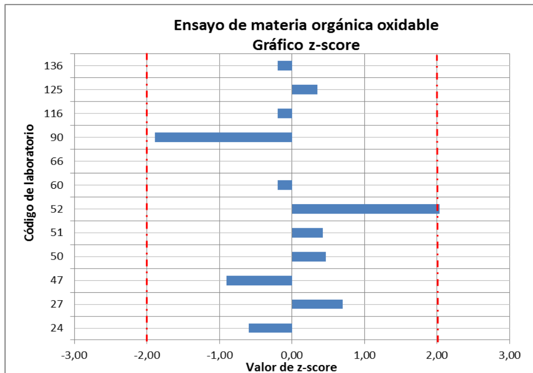
Gráfico 19. Valores de z-score del ensayo de materia orgánica oxidable de suelo por laboratorio a nivel de comunidad autónoma
