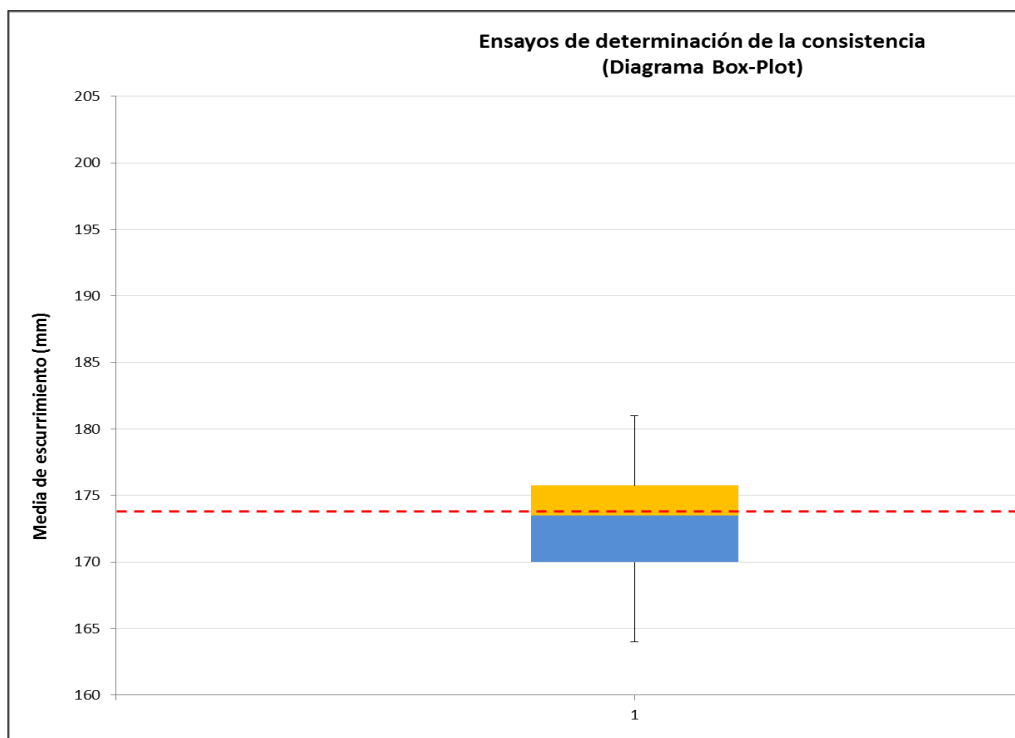
Gráfico 22. Diagrama de cajas y bigotes del ensayo de determinación de la consistencia del mortero a nivel comunidad autónoma
