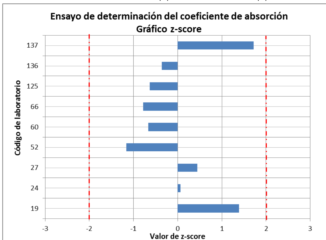
Gráfico 27. Valores de z-score del ensayo de la determinación del coeficiente de absorción del mortero por laboratorio a nivel de comunidad autónoma
