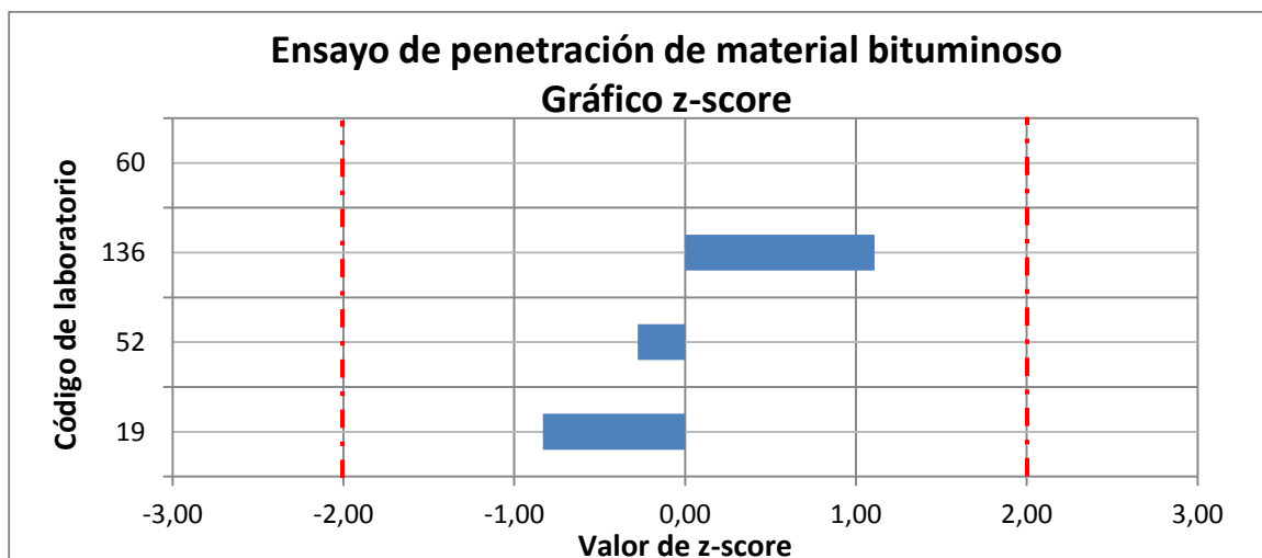
Gráfico 11. Valores de z-score del ensayo de penetración de material bituminoso por laboratorio a nivel de comunidad autónoma
