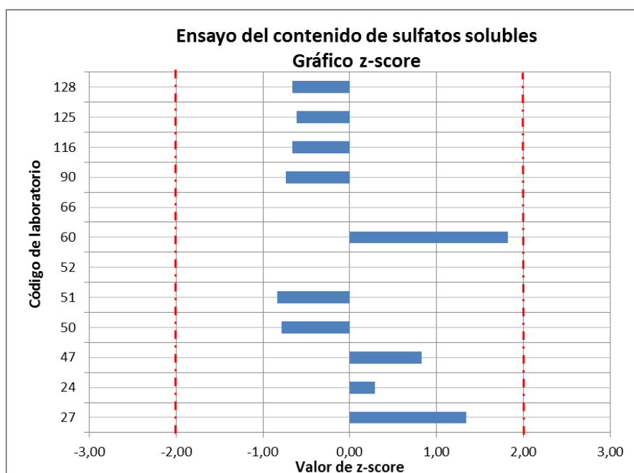
Gráfico 21. Valores de z-score del ensayo de contenido en sulfatos solubles de suelo por laboratorio a nivel de comunidad autónoma
