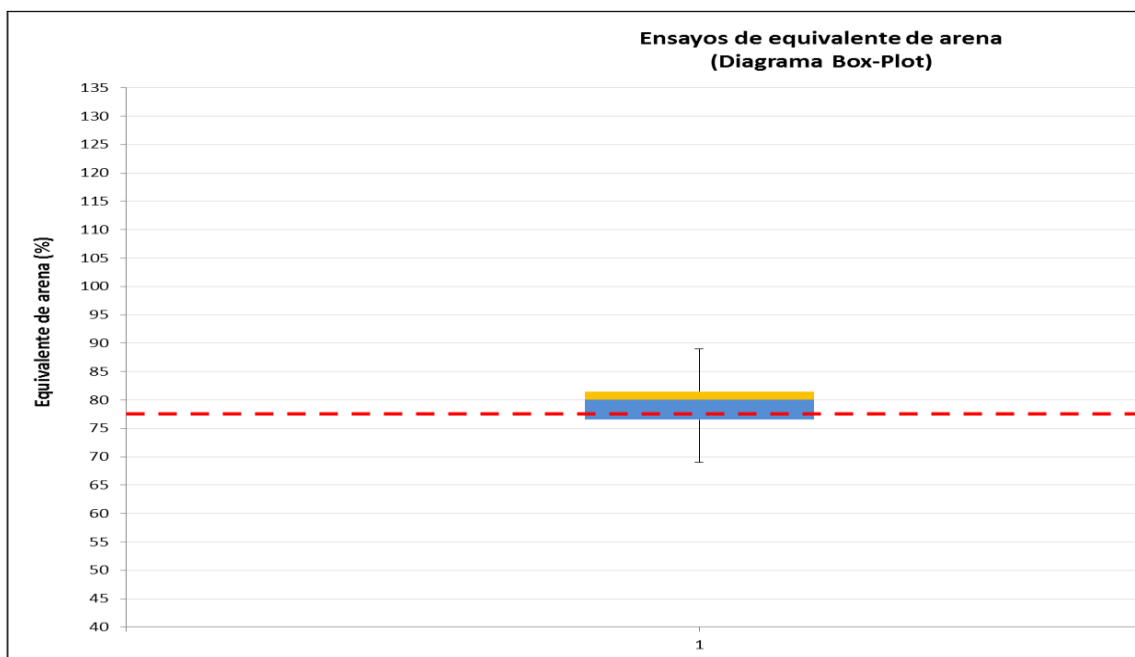
Gráfico 7. Diagrama de cajas y bigotes del ensayo de equivalente de arena de cada Comunidad Autónoma
