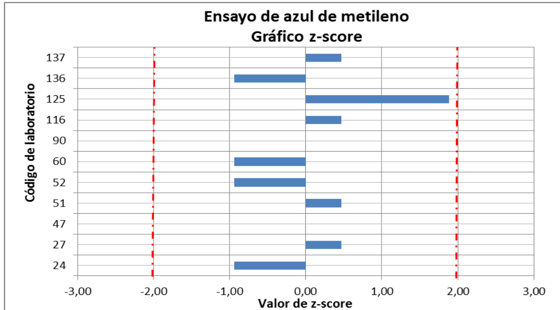
Gráfico 9. Valores de z-score del ensayo de azul de metileno por laboratorio a nivel de comunidad autónoma
