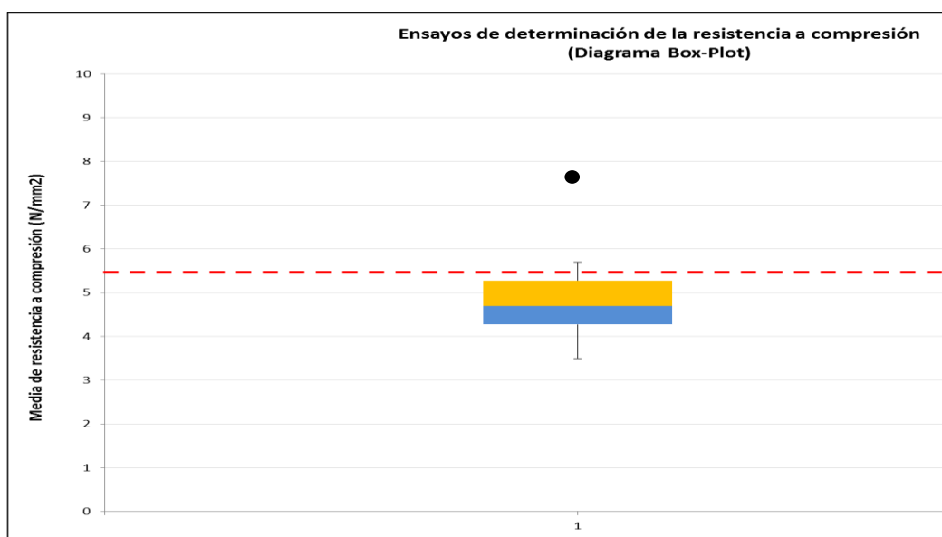
Gráfico. Diagrama de cajas y bigotes del ensayo de determinación de la resistencia a compresión del mortero a nivel comunidad autónoma
