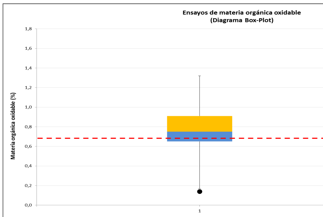
Gráfico 18. Diagrama de cajas y bigotes del ensayo de materia orgánica oxidable en suelo a nivel comunidad autónoma
