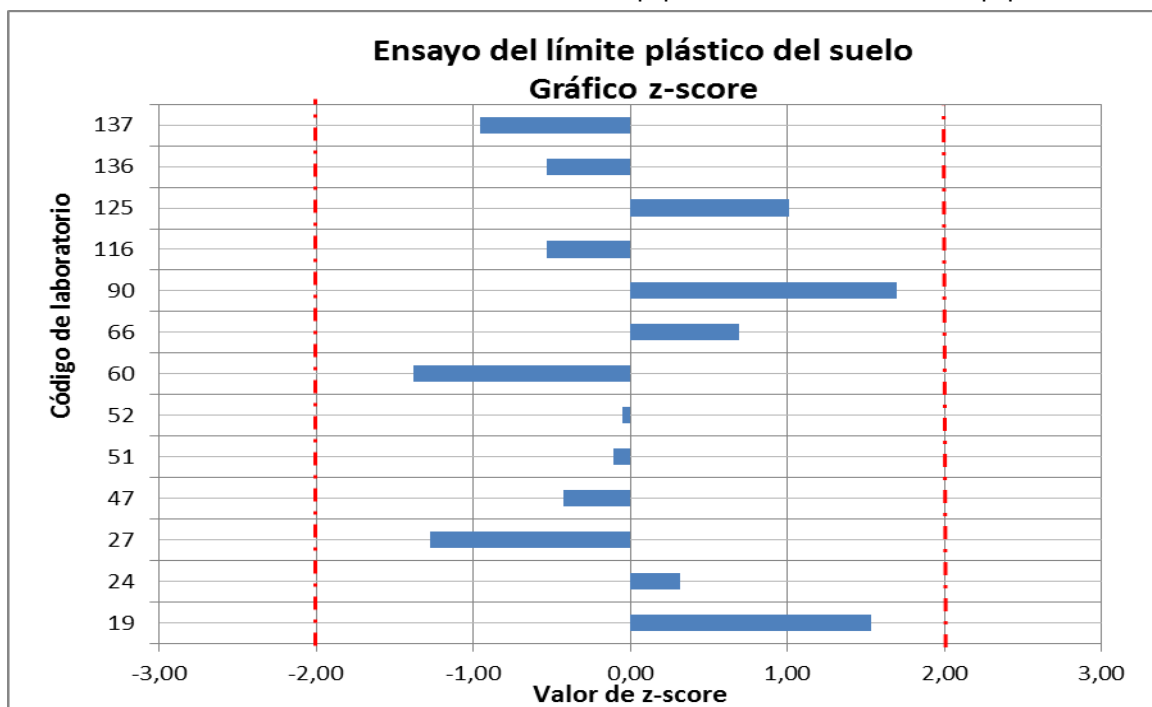
Gráfico 16. Valores de z-score del ensayo de límite plástico de suelo por laboratorio a nivel de comunidad autónoma
