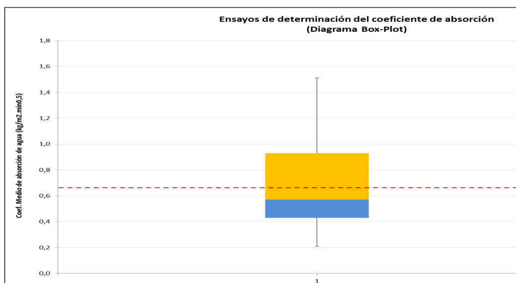
Gráfico. Diagrama de cajas y bigotes del ensayo de determinación del coeficiente de absorción del mortero a nivel comunidad autónoma
