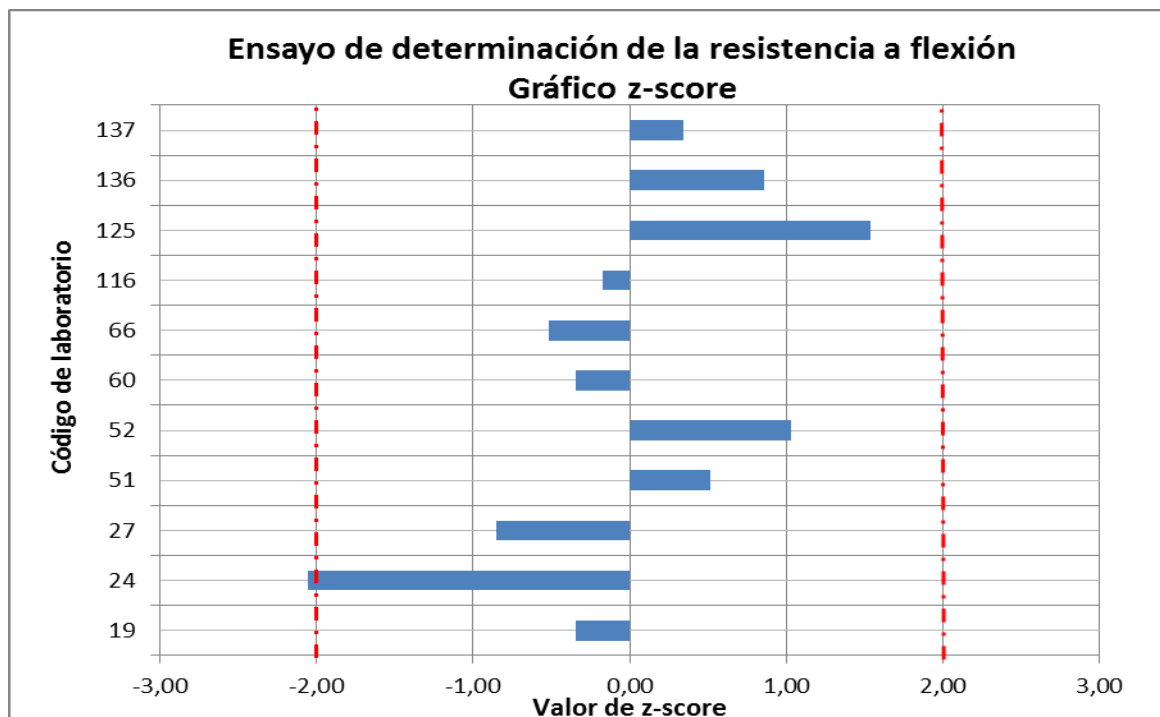
Gráfico 25. Valores de z-score del ensayo de la determinación de la resistencia a flexión del mortero por laboratorio a nivel de comunidad autónoma
