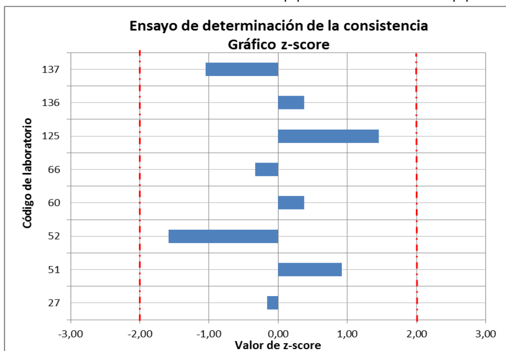
Gráfico 23. Valores de z-score del ensayo de consistencia del mortero por laboratorio a nivel de comunidad autónoma
