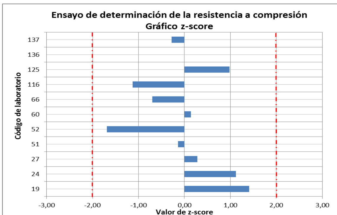
Gráfico 26. Valores de z-score del ensayo de la determinación de la resistencia a compresión del mortero por laboratorio a nivel de comunidad autónoma
