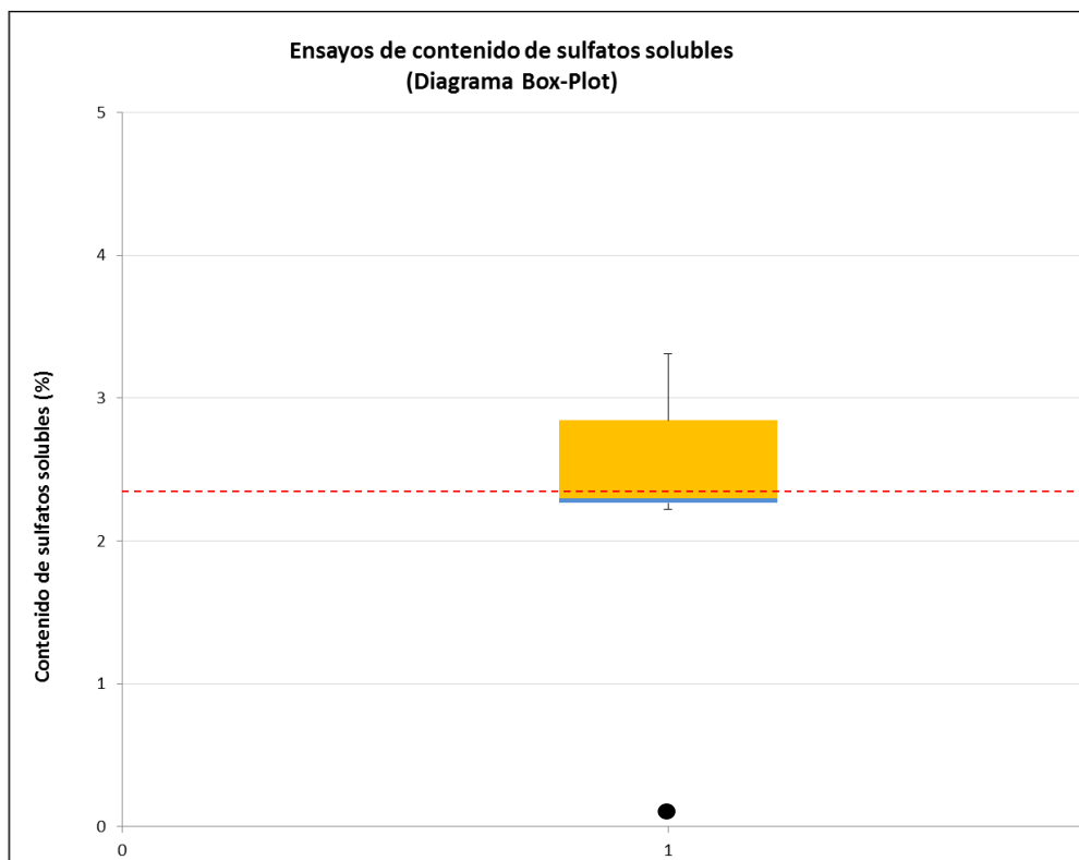
Gráfico 20-. Diagrama de cajas y bigotes del ensayo del contenido en sulfatos solubles en suelo a nivel comunidad autónoma
