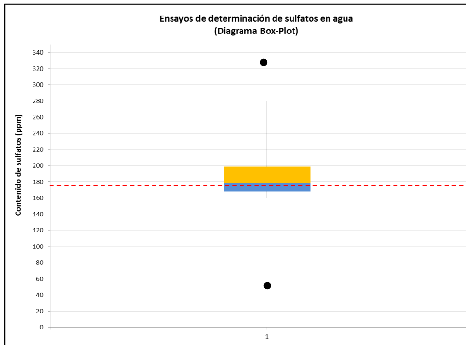
Gráfico 3. Diagrama de cajas y bigotes del ensayo de determinación de sulfatos en agua a nivel de comunidad autónoma
