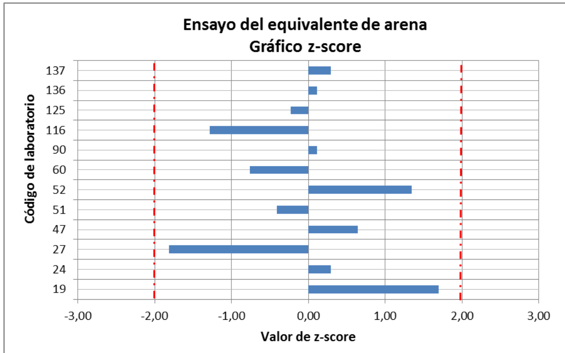
Gráfico 8. Valores de z-score del ensayo de equivalente de arena por laboratorio a nivel de comunidad autónoma
