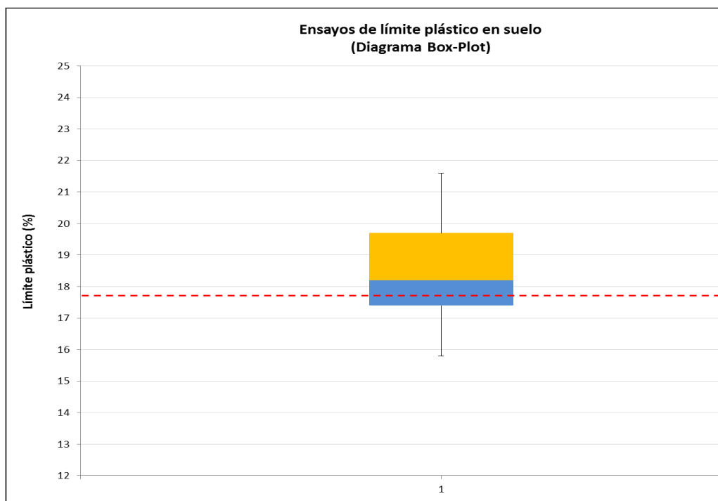
Gráfico 14. Diagrama de cajas y bigotes del ensayo del límite plástico en suelo a nivel comunidad autónoma
