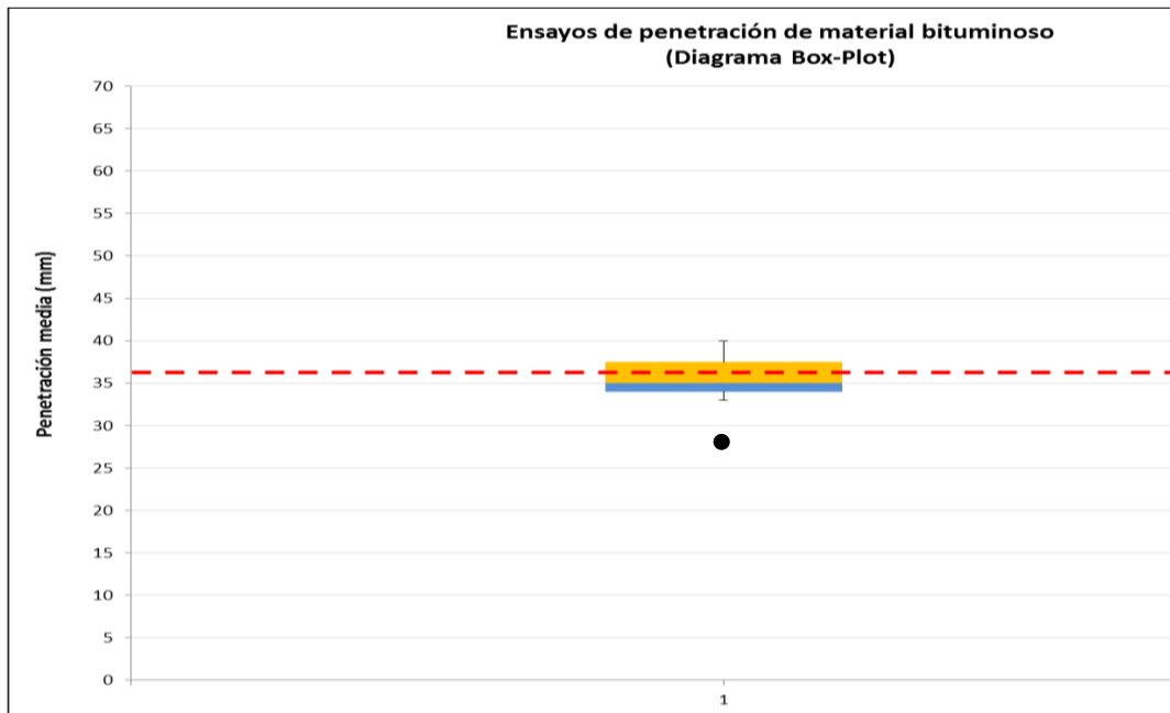
Gráfico 10. Diagrama de cajas y bigotes del ensayo de penetración de material bituminoso a nivel comunidad autónoma
