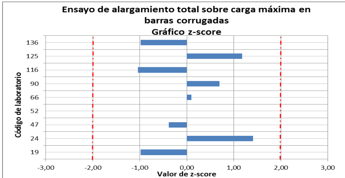
Gráfico 6. Valores de z-score del ensayo de alargamiento total sobre carga máxima en barras corrugadas por laboratorio a nivel de comunidad autónoma
