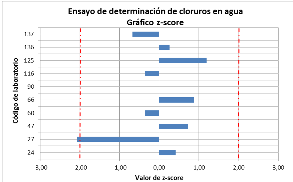
Gráfico 2. Valores de z-score de la determinación de cloruros en agua por laboratorio a nivel de comunidad autónoma.
