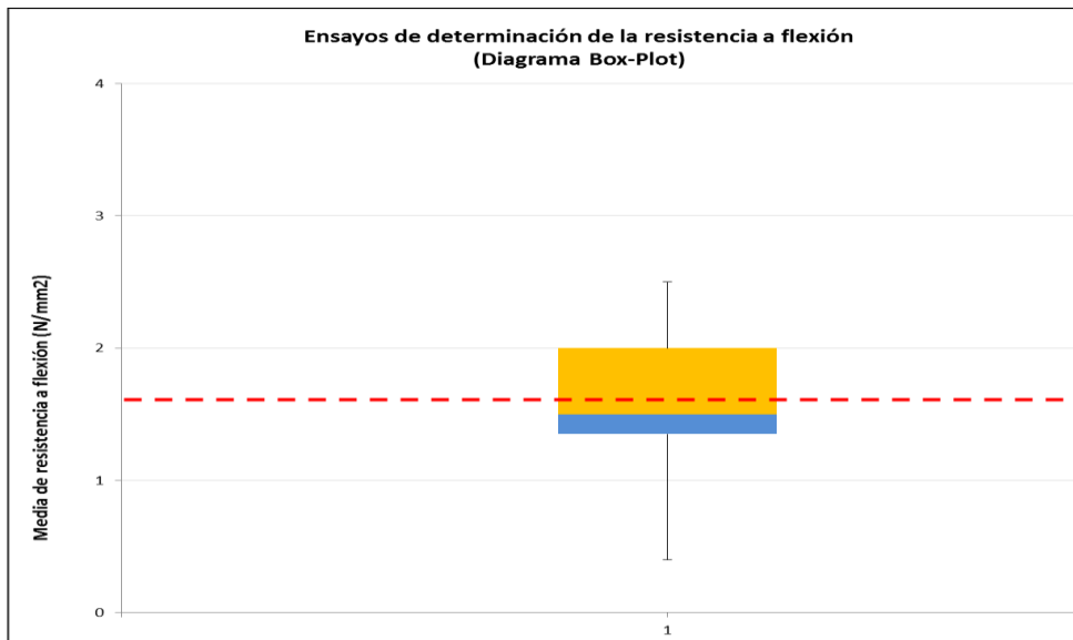
Gráfico 24. Diagrama de cajas y bigotes del ensayo de resistencia a flexión del mortero a nivel comunidad autónoma
