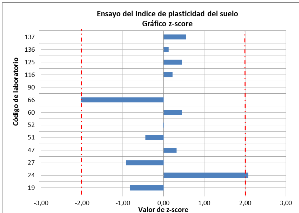
Gráfico 17. Valores de z-score del ensayo de índice de plasticidad de suelo por laboratorio a nivel de comunidad autónoma
