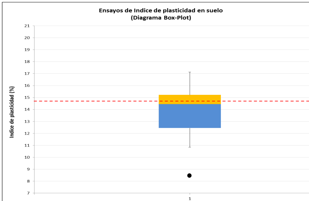
Gráfico 15. Diagrama de cajas y bigotes del ensayo del índice de plasticidad a nivel comunidad autónoma
