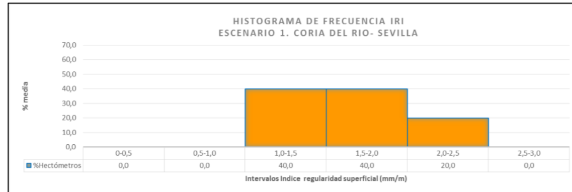
Figura 26. Histograma de frecuencia IRI A-8058 (Sentido Coria del Rio a Sevilla)
