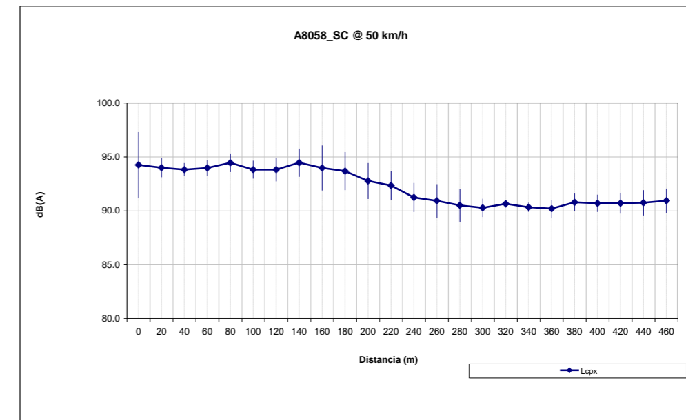
Figura 12 A-8058, 50 km/h en sentido Sevilla Coria
