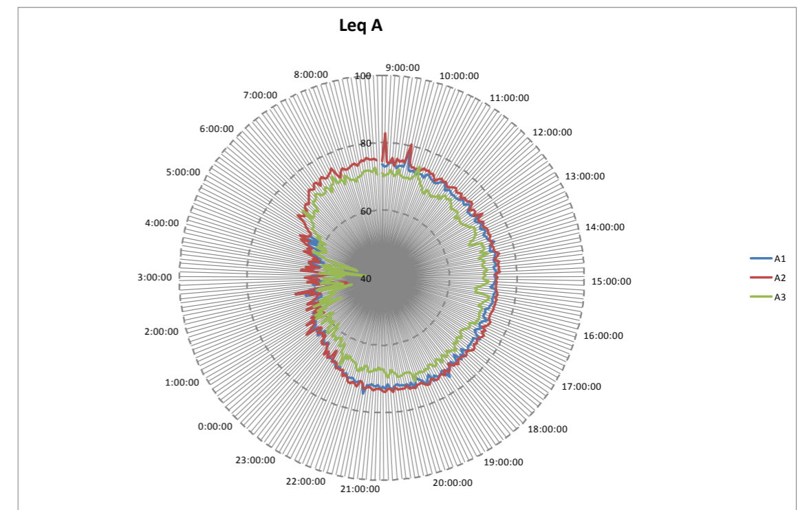
Figura 7. Resultados de Leq (5min) medidos en las estaciones (A1, A2, y A3) en la carretera A-8058.
