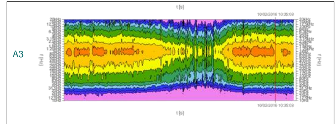
Figura 9. Resultados espectrales de las medidas recogidas por la estación A3 en el escenario 1-B en la carretera A-8058.
