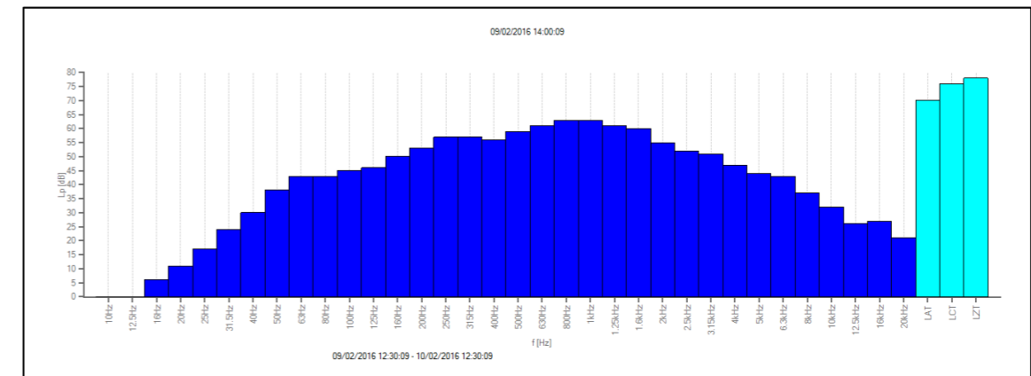
Figura 10. Espectro promedio en tercios de octava de las medidas recogidas por la estación A3 en la carretera A-8058.
