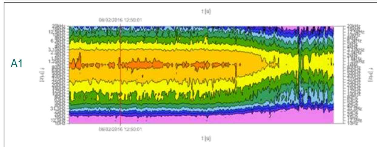
Figura 8. Resultados espectrales de las medidas recogidas por la estación en el escenario 1-A en la carretera A-8058.
