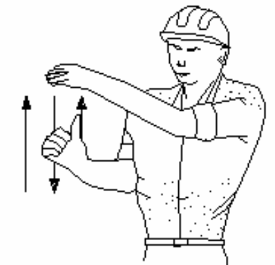
4 LEVANTAR EL AGUJÓN O PLUNA LENTAMENTE
