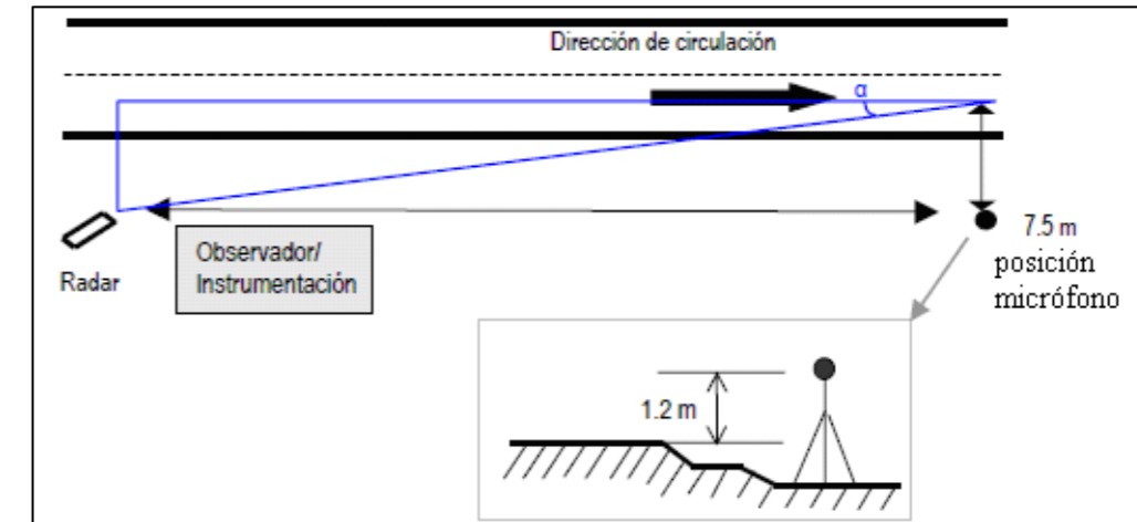
Figura 15. Posicionamiento de los sensores en el ensayo SPB
