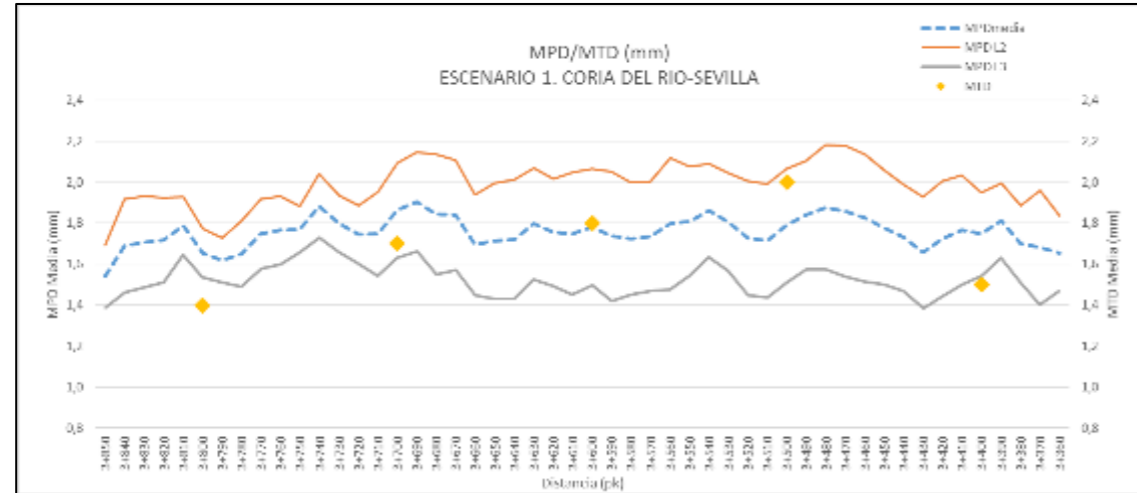
Figura 22. MPD/MTD Escenario 1. Sentido Coria del Rio-Sevilla
