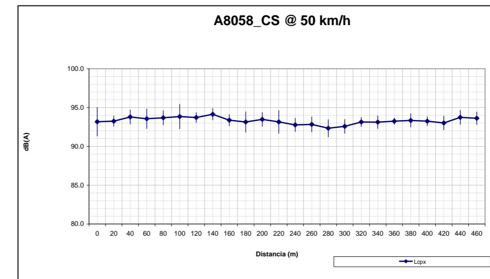
Figura 13: A-8058 a 50 km/h en sentido Coria Sevilla
