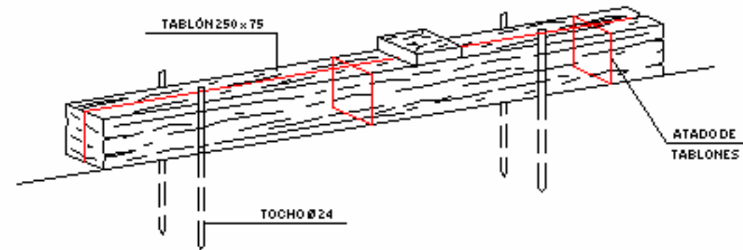
DETALLE DEL CALZO
