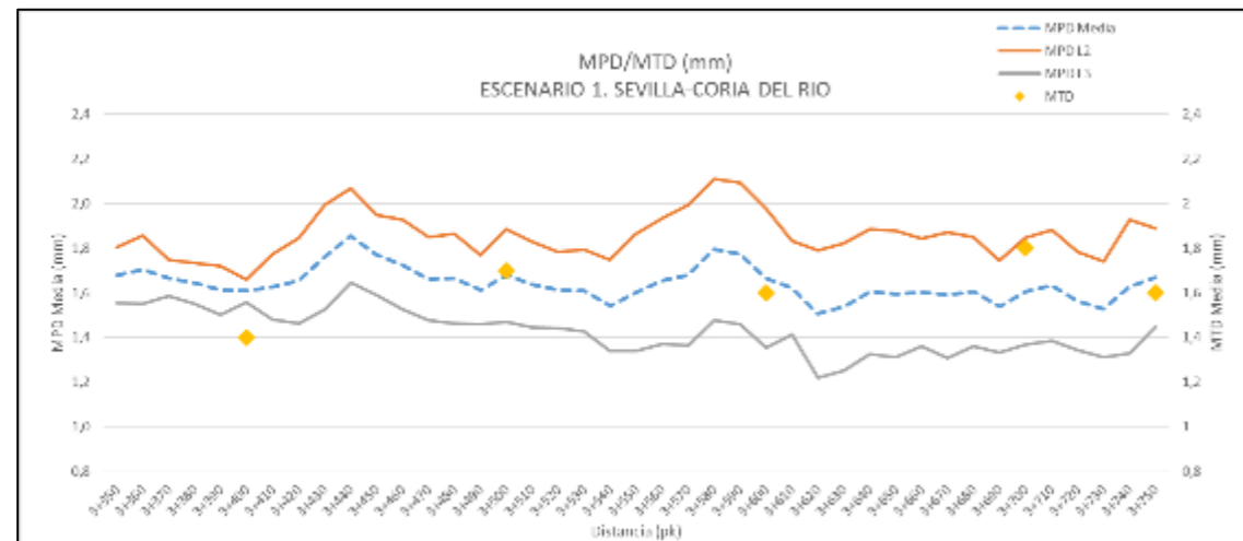
Figura 23. MPD/MTD. Escenario 1. Sentido Sevilla-Coria del Rio
