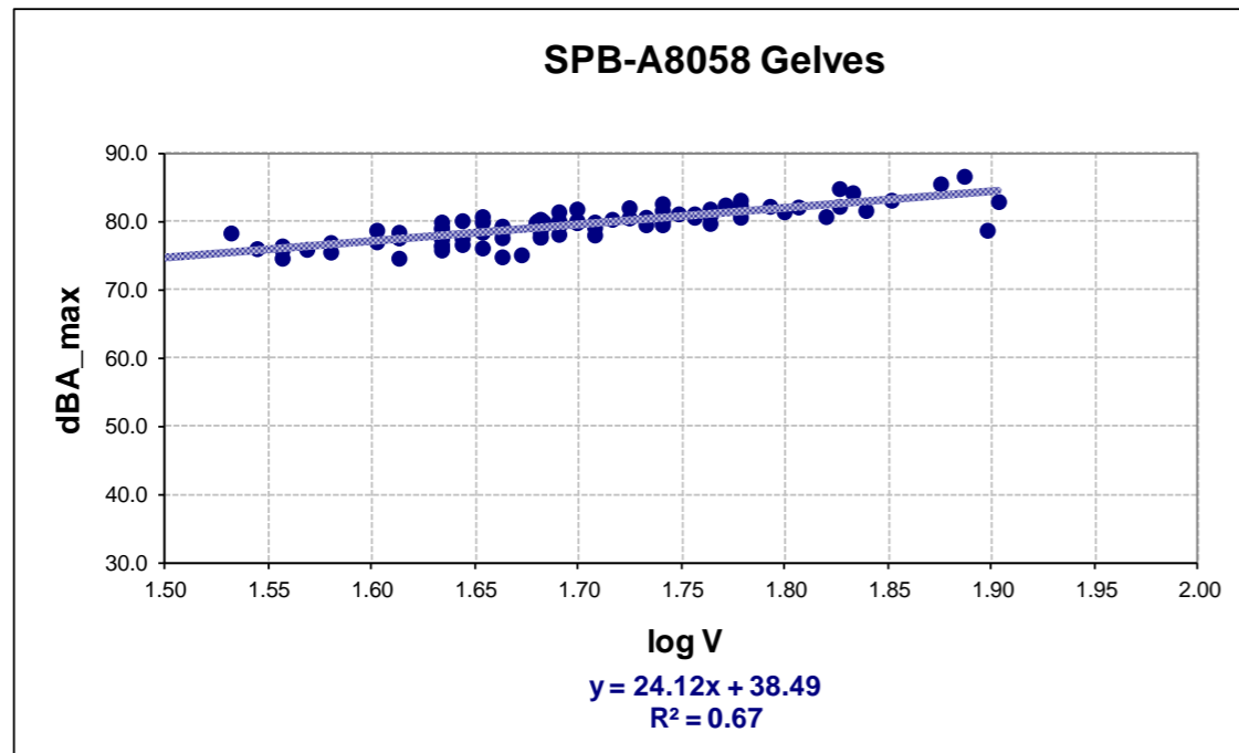
Figura18: Resultados del ensayo SPB A-8058 con velocidad de referencia 50 km/h
