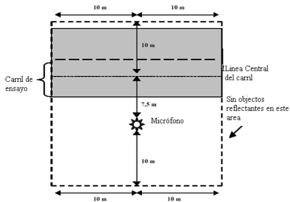
Figura 14. Requerimientos relativos a la ubicación del lugar de ensayo
