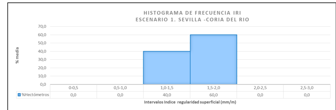
Figura 25. Histograma de frecuencia IRI A-8058 (Sentido Sevilla a Coria del Rio)
