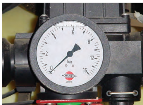
Figura 11. Manómetro logarítmico
