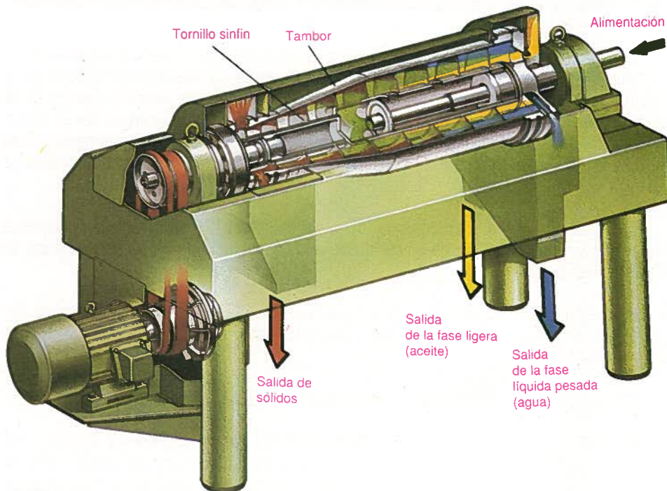
Gráfico 3.- Esquema del decánter de tres fases
