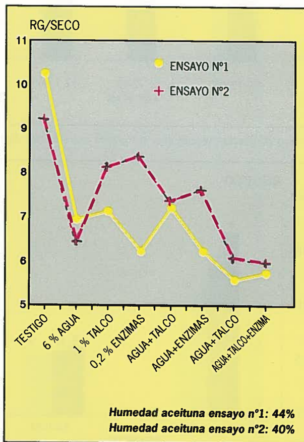
Gráfico 27.- Efecto adición talco, agua y enzimas en Rg/seco orujos de 2 fases. Campaña 93/94.
