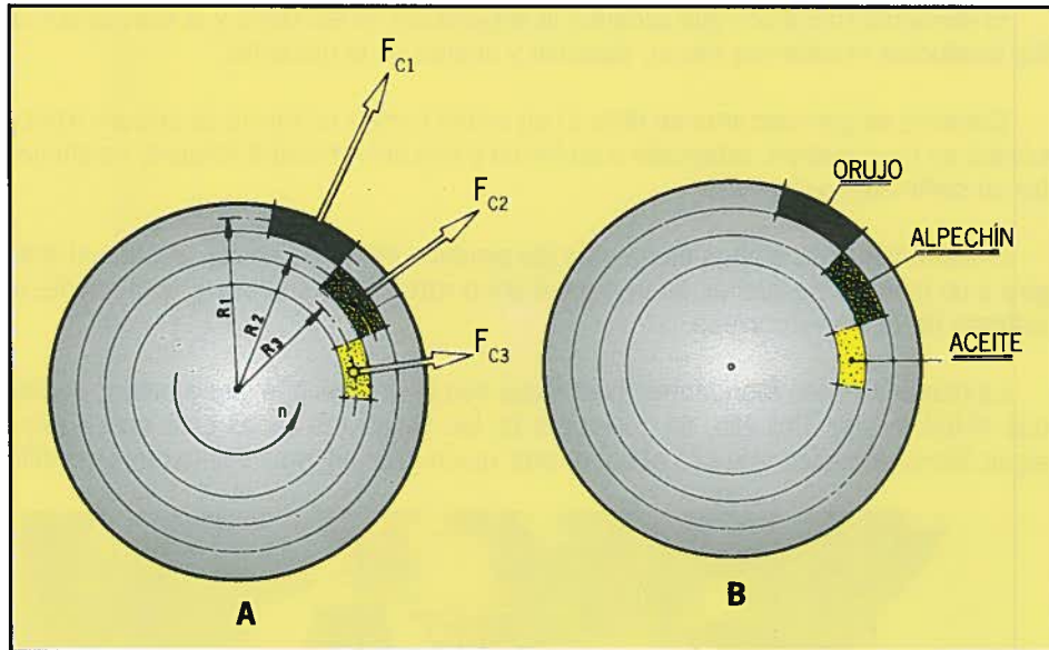
Gráfico 1. Separación en 3 partes (fases), aceite, alpechin y orujo, en la centrífugadora horizontal debido a la fuerza de giro de la misma.
