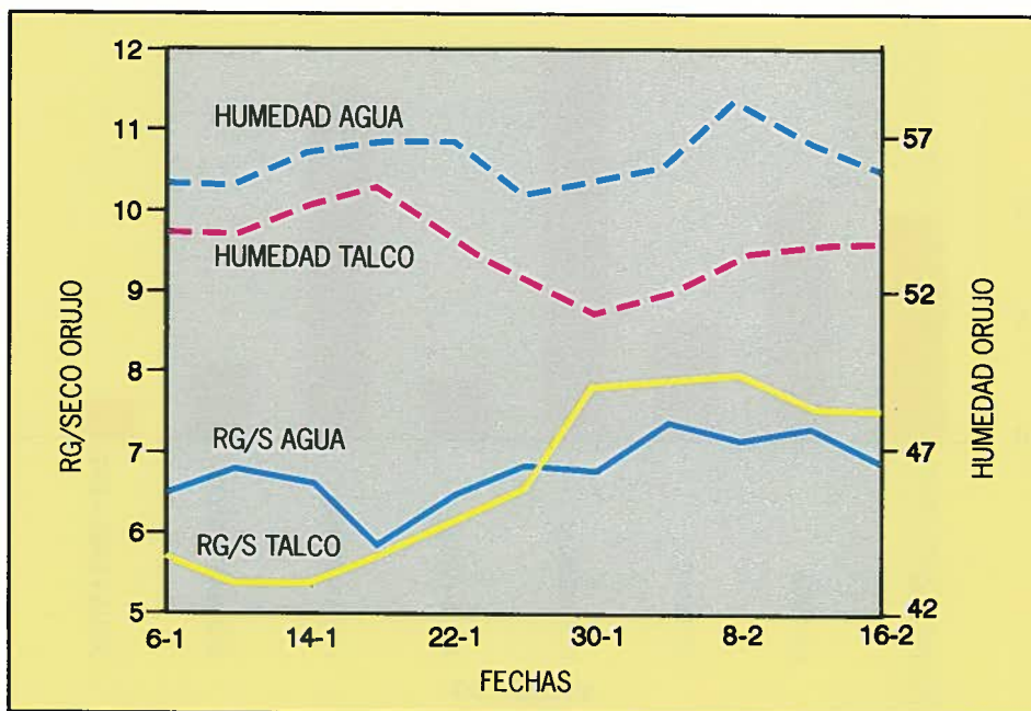
Gráfico 29.- Comparación efecto adición talco o agua en almazaras. Campaña 93/94.
