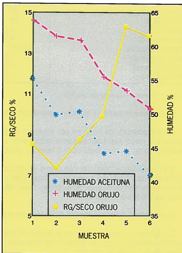
Gráfico 8.- Relación entre humedad (aceituna y orujo) y Rg/seco orujo 2 fases.
