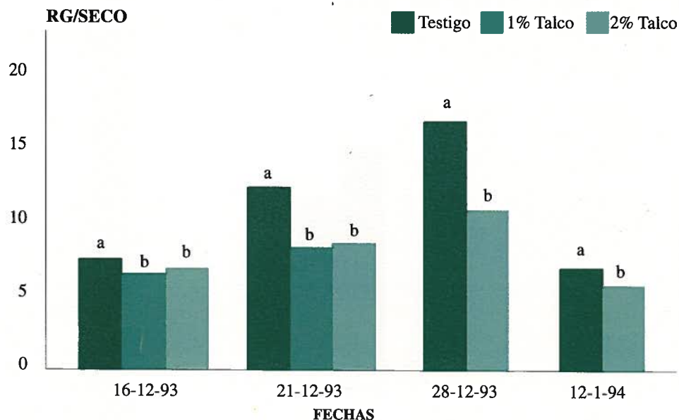
Gráfico 22.- Efecto adición talco en el Rg/seco orujos de 2 fases. Campaña 93/94.
