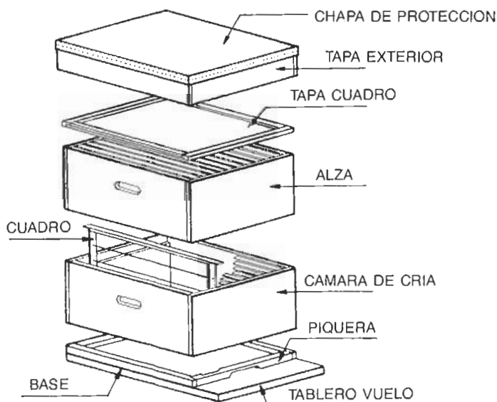
Figura nº 23: COLMENA LANGSTROTH (despiece por elementos, en perspectiva)
