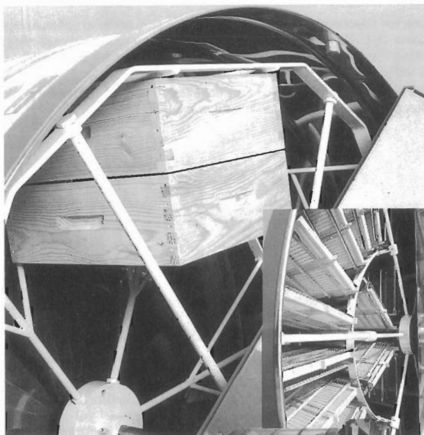
Foto n.º 12: Extractor radial, de gran capacidad para explotaciones industriales
