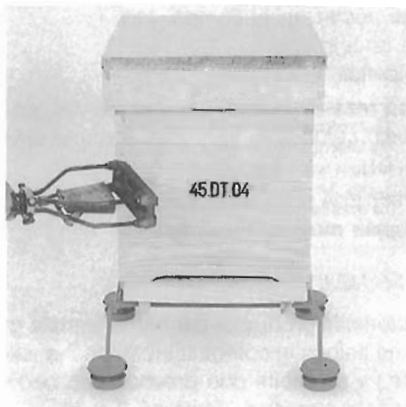
Foto n.º 5: Marcador de colmenas
