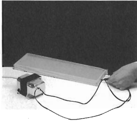
Foto n.º 8: Fijación de la lámina de cera al cuadro
