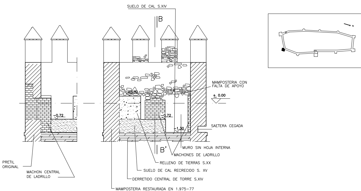
SECCION B-B'
