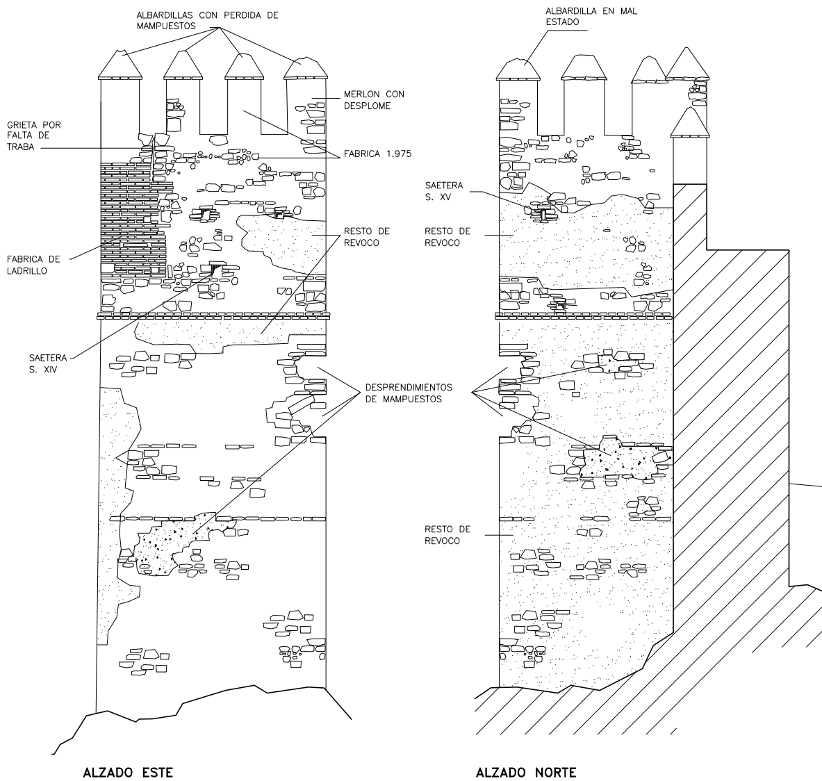
ALZADO ESTE
