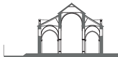
Sección transversal
