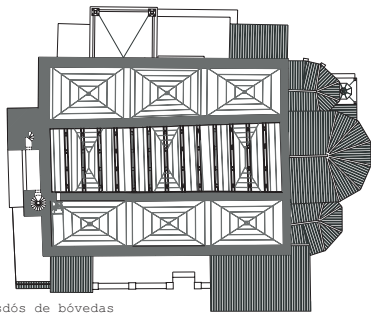
Planta de trasdós de bóvedas
