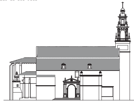
Alzado del Evangelio
