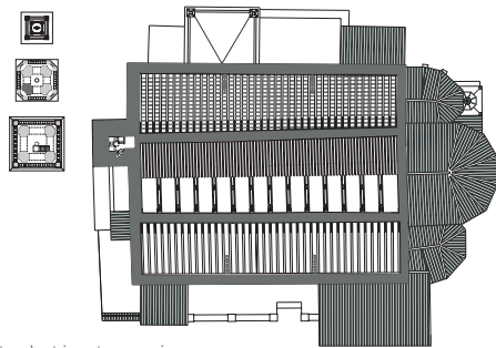
Planta de tirantes y vigas
