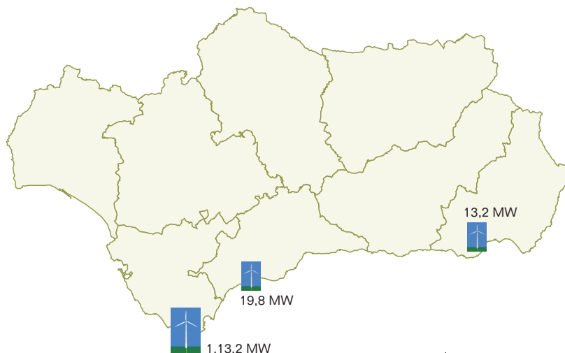
Potencia eléctrica instalada en parques eólicos en Andalucía en el año 2000
