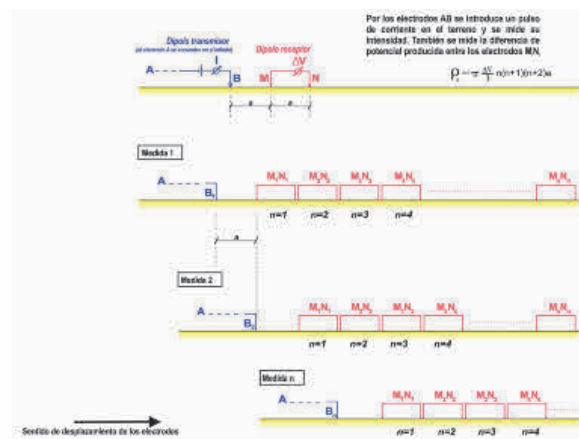
Figura 13. Dispositivo tipo Polo-Dipolo empleado para las medidas de resistividad aparente del terreno.
