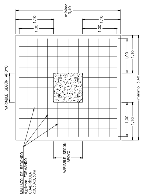
PLANTA MALLA EQUIPOTENCIAL
