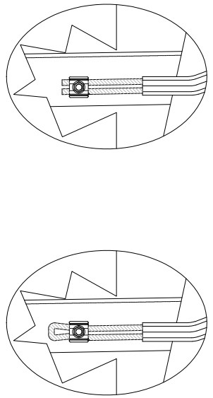
DETALLE DE CONEXION DEL ANILLO A LA ESTRUCTURA DEL APOYO
