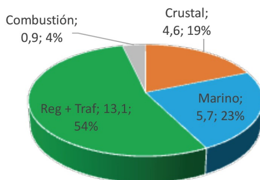
Figura 6.24. Contribución de fuentes en el periodo 2021 para PM_{10} en la estación de Plaza del Castillo
