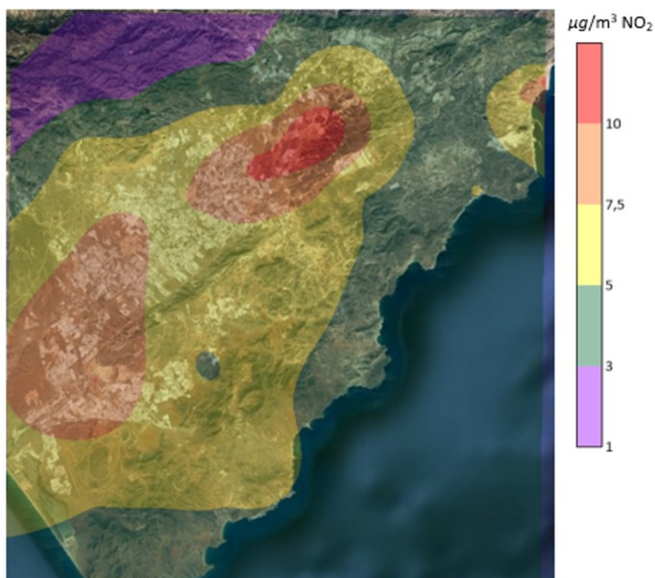
Figura 5.24. Resultados de la campaña de captadores difusivos de \text{NO}_2 ( \mu\text{g}/\text{m}^3 ) en la Zona Industrial de Carboneras
