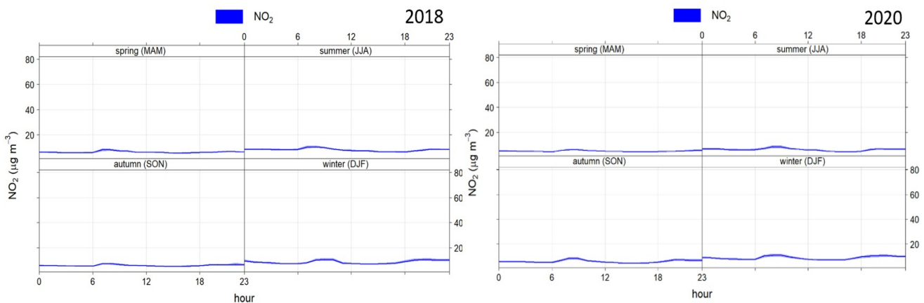
Figura 6.12. Patrón horario estacional para NO 2 en 2018 y 2020. Estación Rodalquilar
