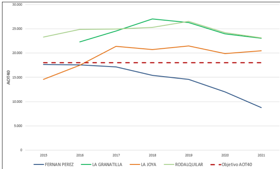
Figura 5.11. AOT40 ( \mu\text{g}/\text{m}^3 \text{ h} ) calculada para Zona industrial de Carboneras
