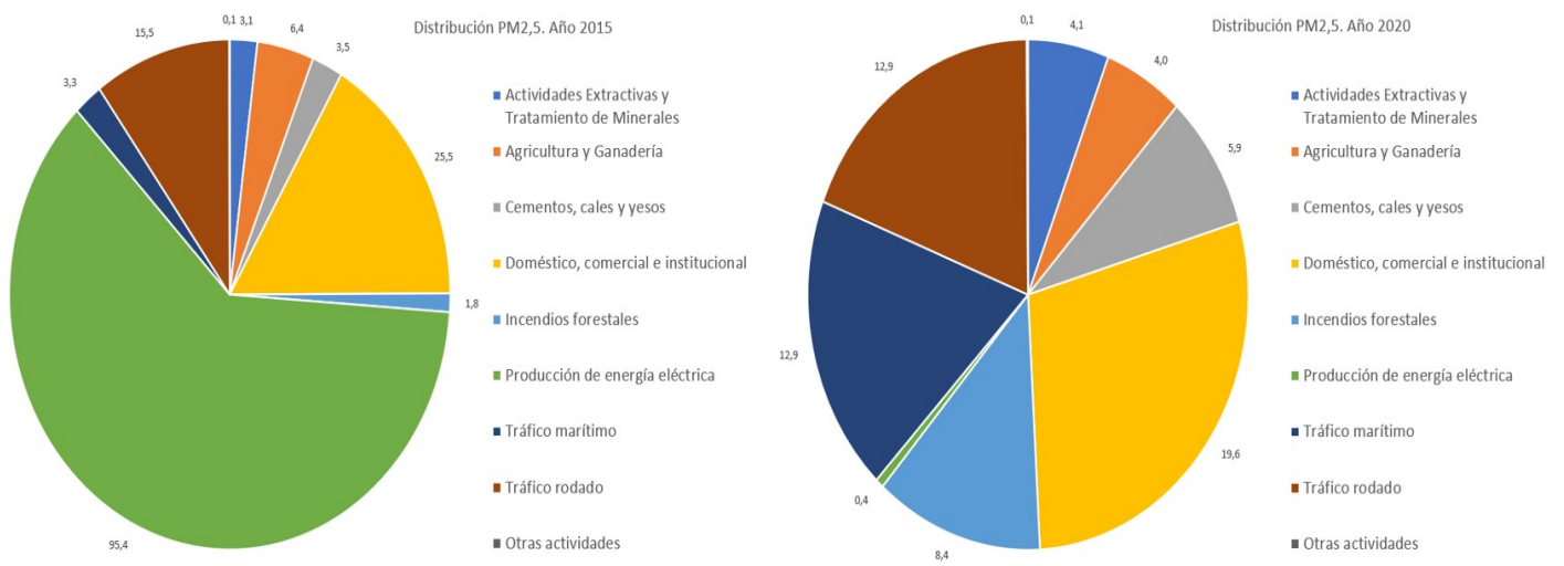
Figura 6.33. Distribución por sectores de las emisiones inventariadas en los años 2015 y 2020 de PM 2,5 (t/año)
