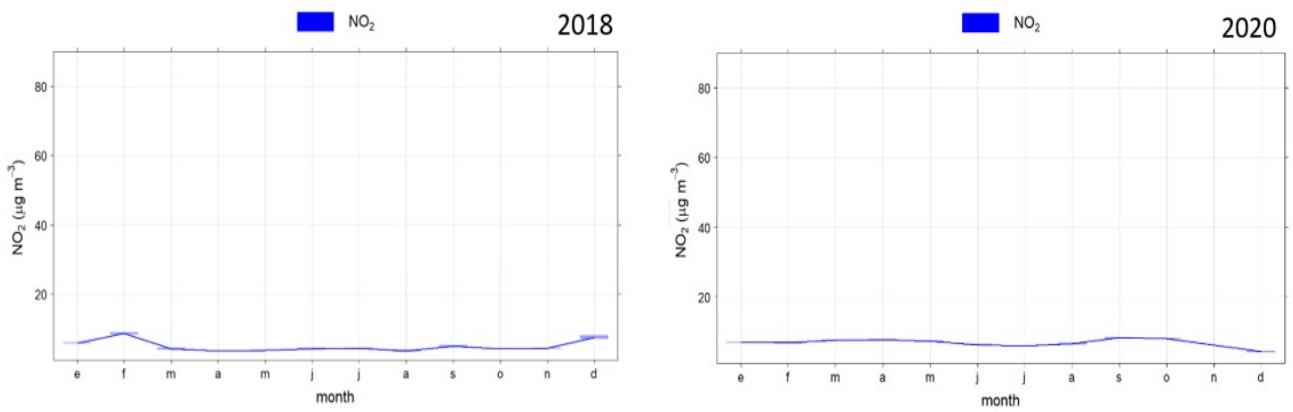
Figura 6.4. Medias mensuales de NO 2 en los años 2018 y 2020. Estación Fernán Pérez
