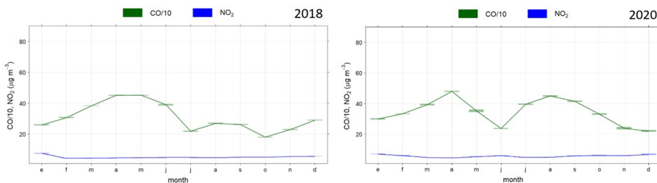
Figura 6.2. Medias mensuales de NO 2 y CO en los años 2018 y 2020. Estación La Joya
