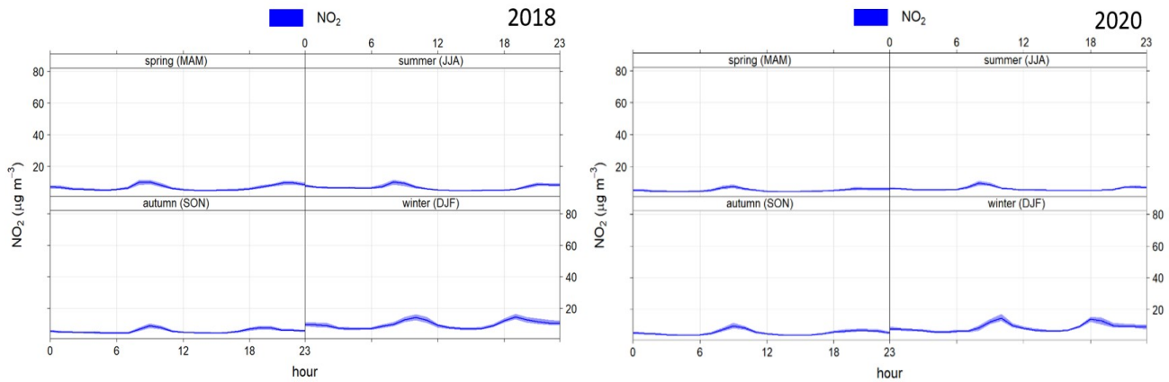
Figura 6.11. Patrón horario estacional para NO 2 en 2018 y 2020. Estación La Granatilla
