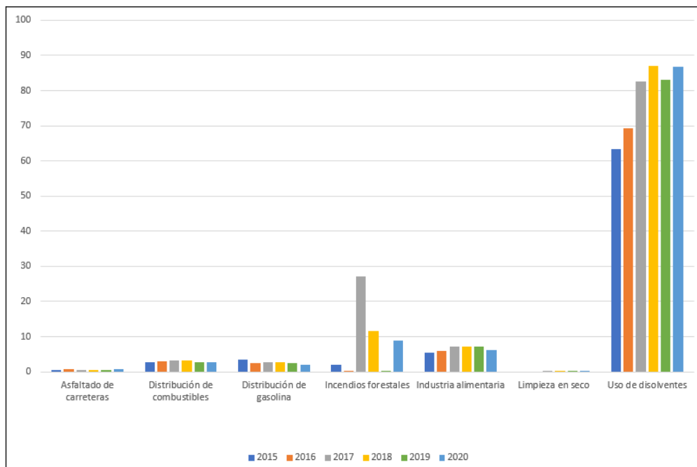
Figura 6.36. Evolución de las emisiones inventariadas de COVNM (t/año) en el grupo “otras actividades”
