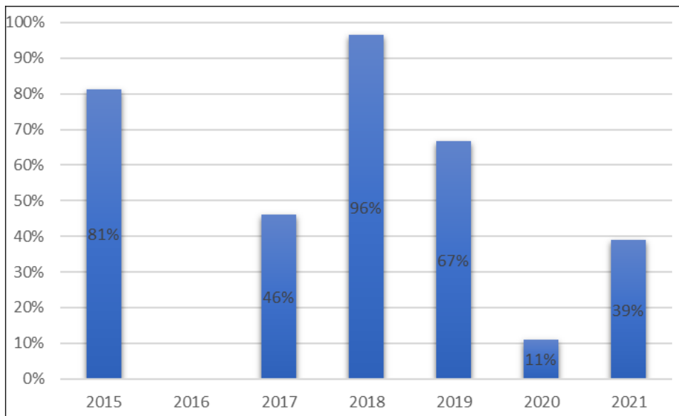
Figura 5.30. Porcentaje de la contribución de los eventos de intrusiones de masas de aire norteafricano al número de superaciones del valor límite diario en Plaza del Castillo
