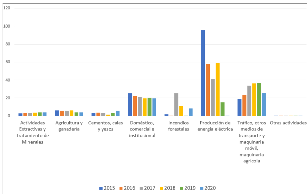
Figura 6.28. Evolución de las emisiones inventariadas de PM 2,5 (t/año)
