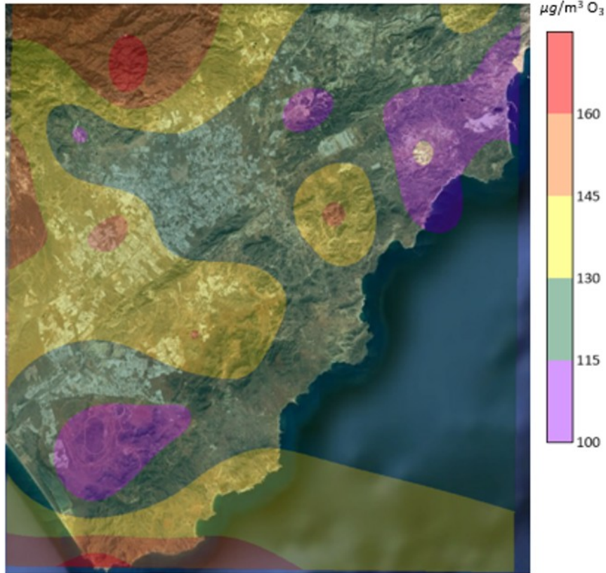
Figura 5.25. Resultados de la campaña de captadores difusivos de O 3 (µg/m 3 ) en la Zona Industrial de Carboneras
