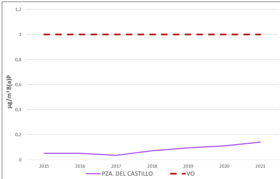
Figura 5.15. Medias anuales de B(a)P (ng/m 3 ) en Zona Industrial de Carboneras
