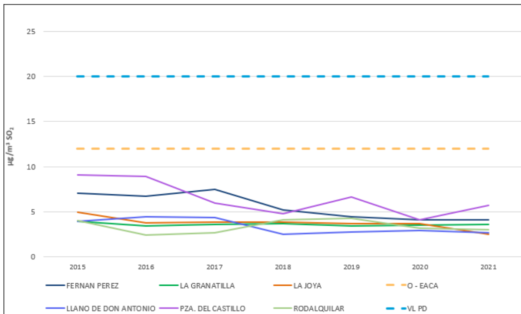
Figura 5.13. Promedio anual de SO 2 ( \mu\text{g}/\text{m}^3 ) frente al futuro valor límite anual (propuesta de directiva de calidad del aire) en Zona Industrial de Carboneras
