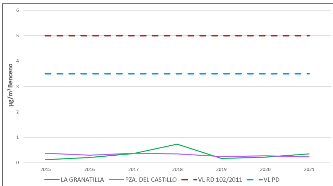
Figura 5.14. Valor límite anual de benceno ( \mu\text{g}/\text{m}^3 ) para la protección de la salud en Zona Industrial de Carboneras
