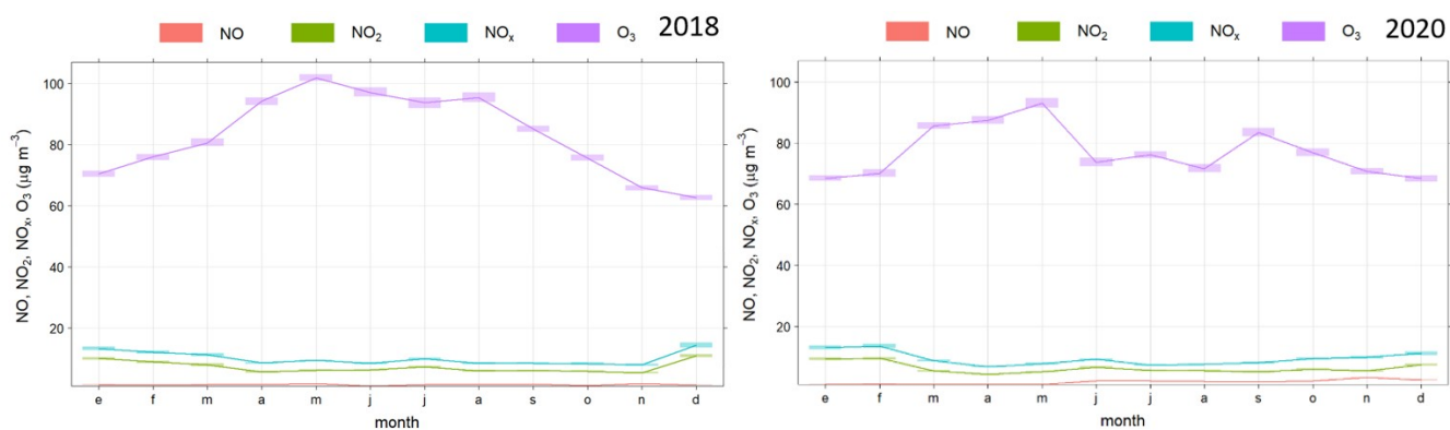
Figura 6.14. Medias mensuales de \text{O}_3 , \text{NO}_x , \text{NO}_2 y \text{NO} en los años 2018 y 2020. Estación La Granatilla
