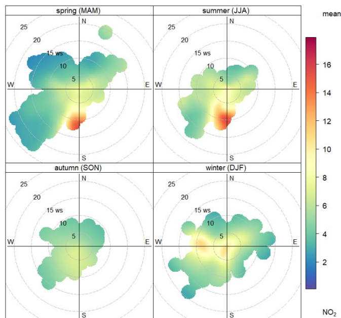
Figura 6.22. Relación entre los niveles horarios de NO 2 y la velocidad y dirección del viento en 2018. Estación Plaza del Castillo
