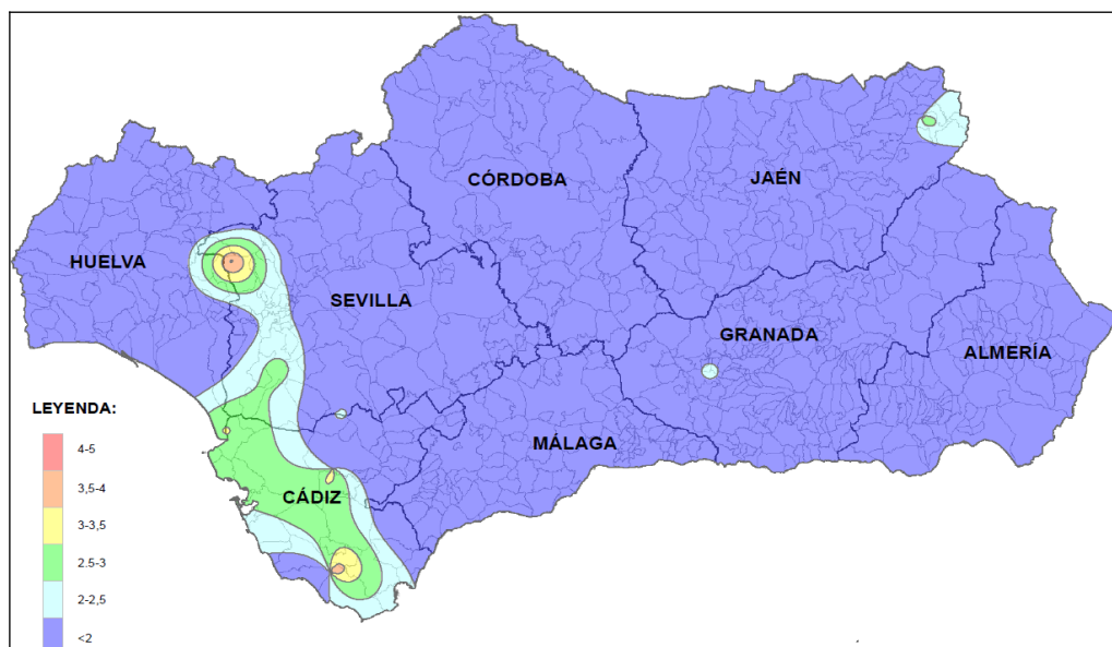
Figura 5.23. Resultados de la campaña de captadores difusivos en fondo rural. Promedio de SO_2 en 2020
