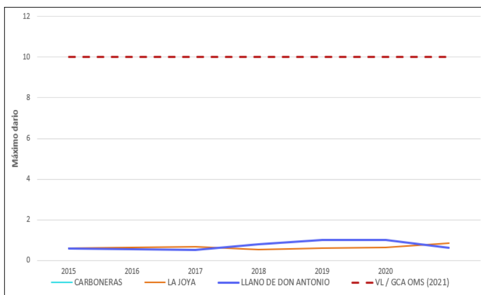
Figura 5.8. Máxima diaria de las medias móviles octohorarias de monóxido de carbono (mg/m 3 ) en Zona Industrial de Carboneras
