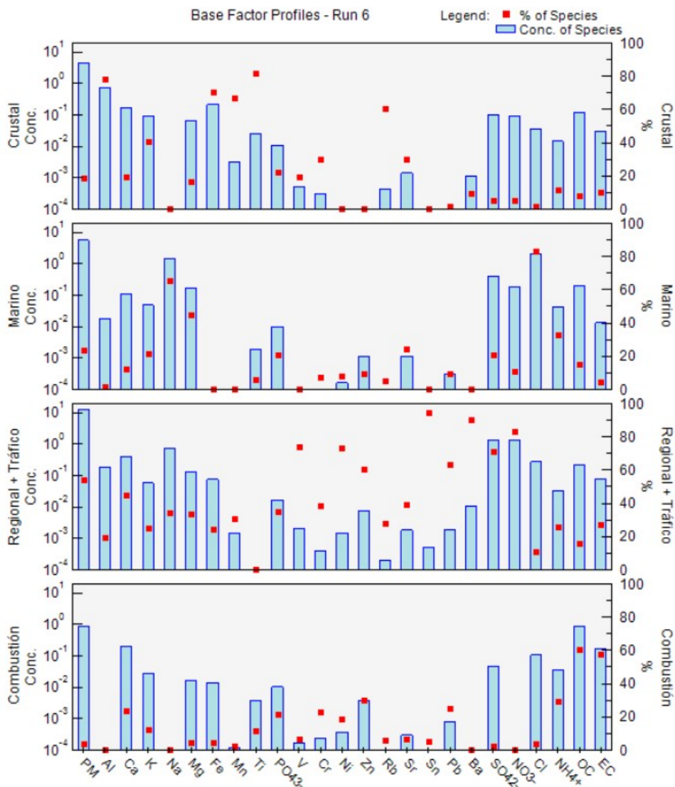
Figura 6.25. Perfil químico de las fuentes de PM 10 (expresado como contribución de elementos mayores y traza en µg/m 3 ) determinadas en la estación de Plaza del Castillo en el año 2021
