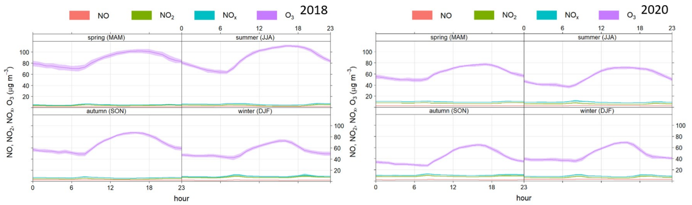
Figura 6.17. Patrón horario estacional para O 3 , NO x , NO 2 y NO en 2018 y 2020. Estación Fernán Pérez
