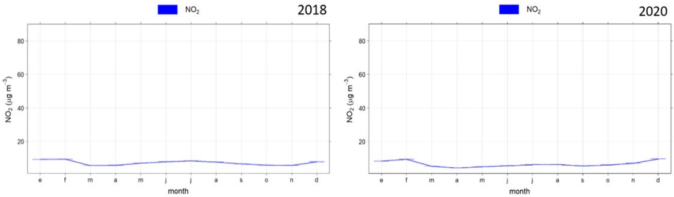
Figura 6.6. Medias mensuales de NO 2 en los años 2018 y 2020. Estación Rodalquilar
