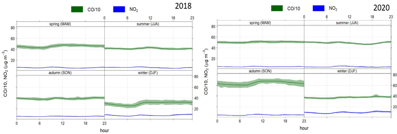
Figura 6.9. Patrón horario estacional para NO 2 y CO en 2018 y 2020. Estación Llano de Don Antonio
