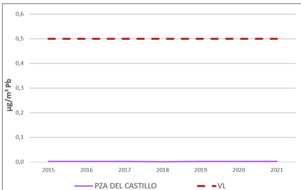
Figura 5.19. Medias anuales de Pb ( \mu\text{g}/\text{m}^3 ) en Zona Industrial de Carboneras
