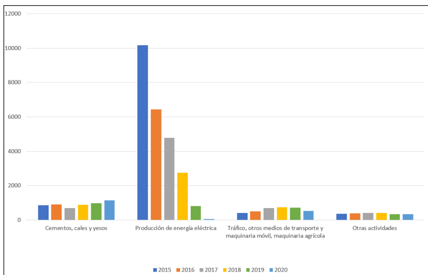
Figura 6.30. Evolución de las emisiones inventariadas de \text{NO}_x (t/año)
