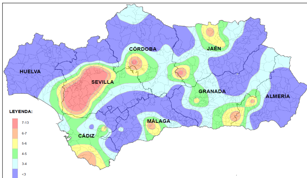
Figura 5.21. Resultados de la campaña de captadores difusivos en fondo rural. Promedio de NO x en 2020
