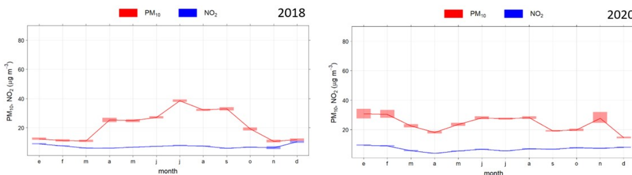
Figura 6.1. Medias mensuales de NO 2 y PM 10 en los años 2018 y 2020. Estación Plaza del Castillo
