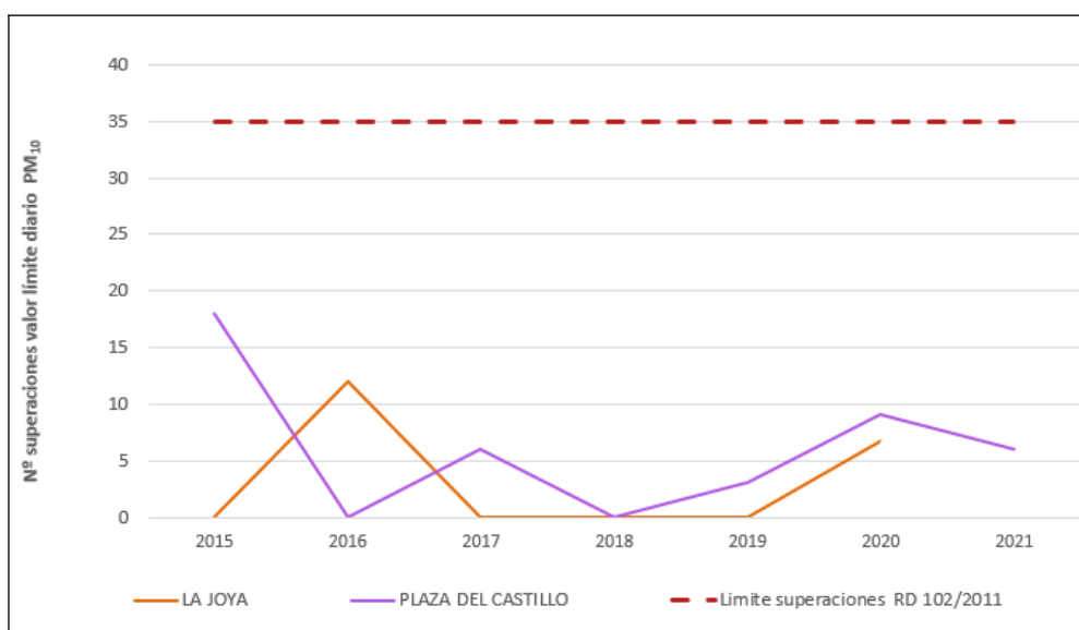
Figura 5.4. Número de superaciones del valor límite diario de PM 10 en Zona Industrial de Carboneras
