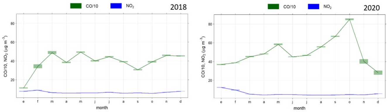
Figura 6.3. Medias mensuales de NO 2 y CO en los años 2018 y 2020. Estación Llano Don Antonio
