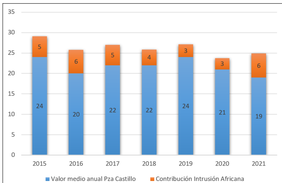
Figura 5.31. Contribución de la carga neta de polvo africano al valor media anual ( \mu g/m^3 ). Estación Plaza del Castillo
