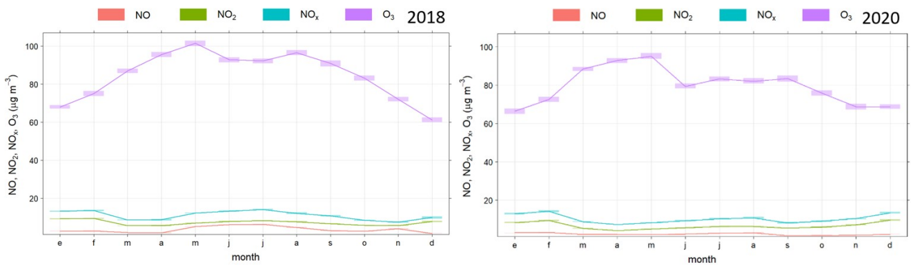
Figura 6.16. Medias mensuales de O 3 , NO x , NO 2 y NO en los años 2018 y 2020. Estación Rodalquilar
