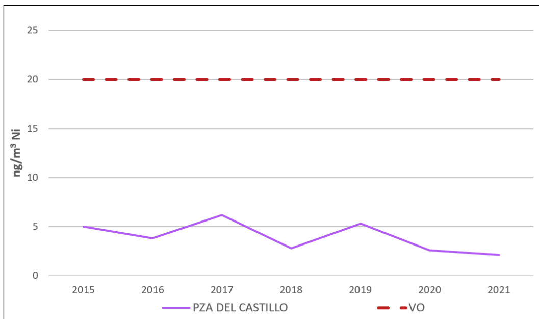
Figura 5.18. Medias anuales de Ni (ng/m³) en Zona Industrial de Carboneras
