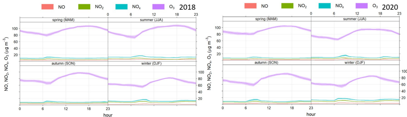
Figura 6.20. Patrón horario estacional para O 3 , NO x , NO 2 y NO en 2018 y 2020. Estación Rodalquilar
