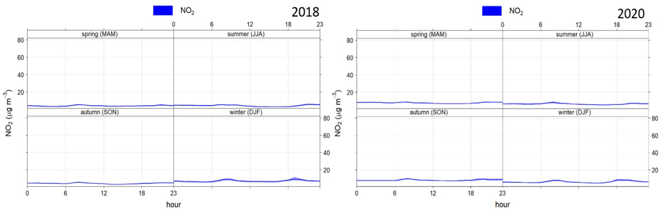
Figura 6.10. Patrón horario estacional para NO 2 en 2018 y 2020. Estación Fernán Pérez
