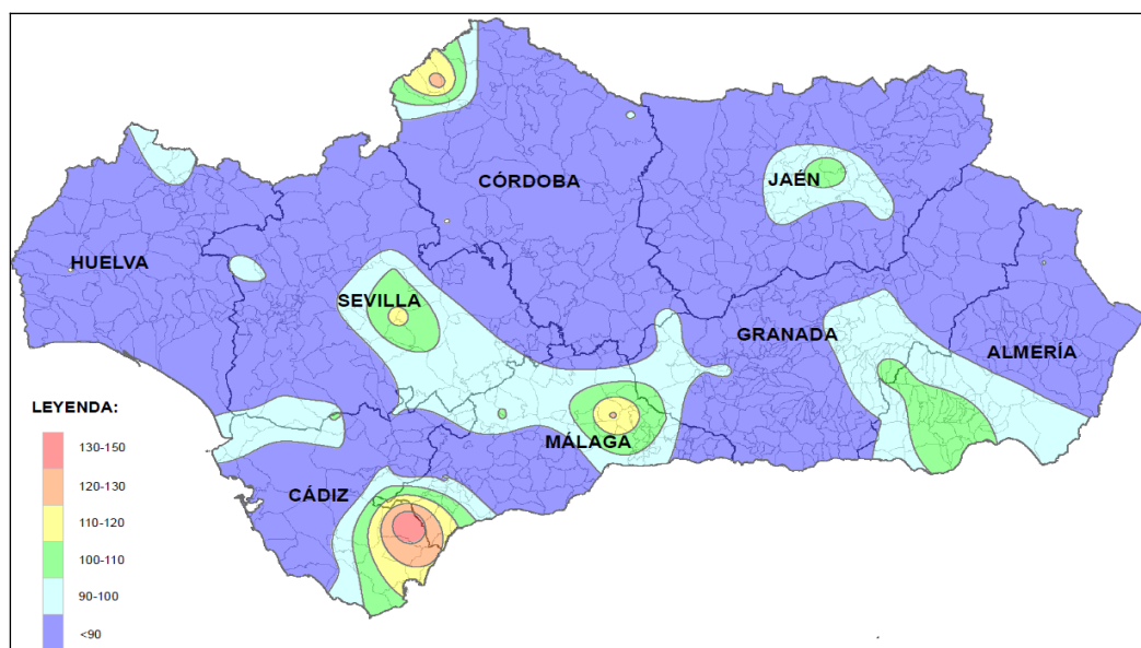
Figura 5.22. Resultados de la campaña de captadores difusivos en fondo rural. Promedio de O_3 en 2020
