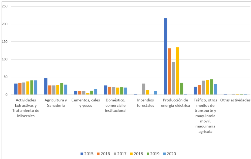
Figura 6.27. Evolución de las emisiones inventariadas de PM 10 (t/año)
