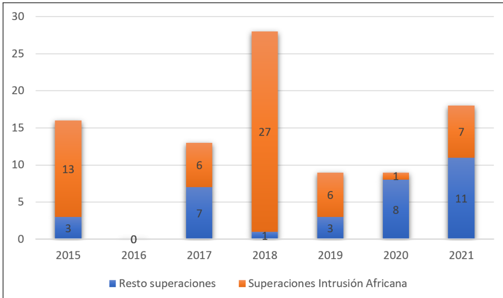
Figura 5.29. Origen y cuantificación del número de superaciones diarias de PM 10 (µg/m 3 ) en la estación Plaza Castillo 1
