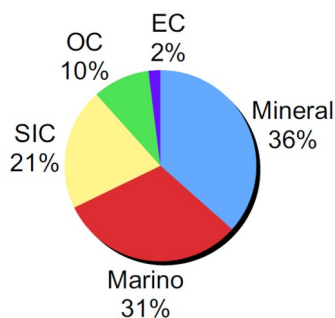
Figura 6.23. Distribución de componentes químicos principales en PM 10 . Estación de Plaza Castillo (Almería)
