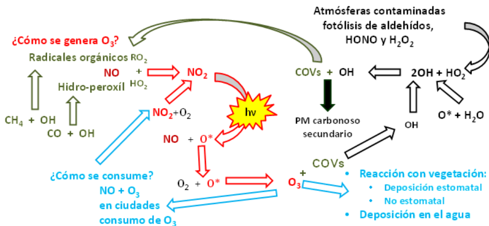
Figura 6.37. Procesos de generación y consumo de O 3
