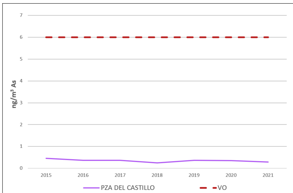
Figura 5.16. Medias anuales de As (ng/m 3 ) en Zona Industrial de Carboneras
