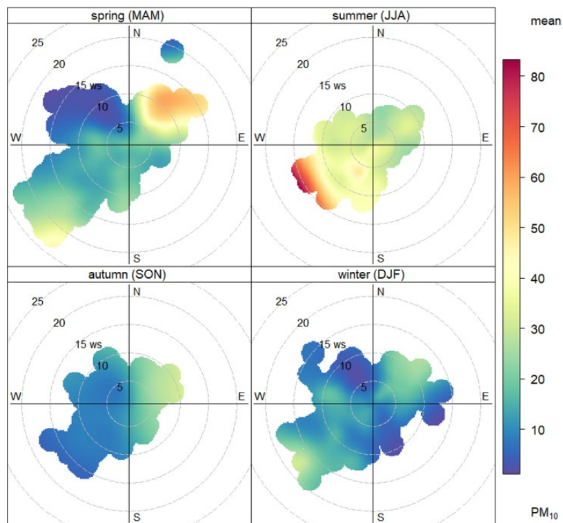
Figura 6.21. Relación entre los niveles horarios de PM 10 y la velocidad y dirección del viento en 2018. Estación Plaza del Castillo
