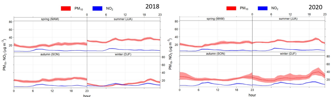
Figura 6.7. Patrón horario estacional para NO 2 y PM 10 en 2018 y 2020. Estación Plaza del Castillo
