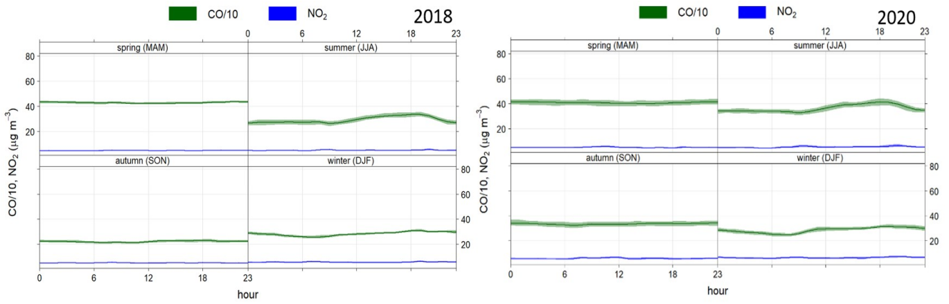
Figura 6.8. Patrón horario estacional para NO 2 y CO en 2018 y 2020. Estación la Joya
