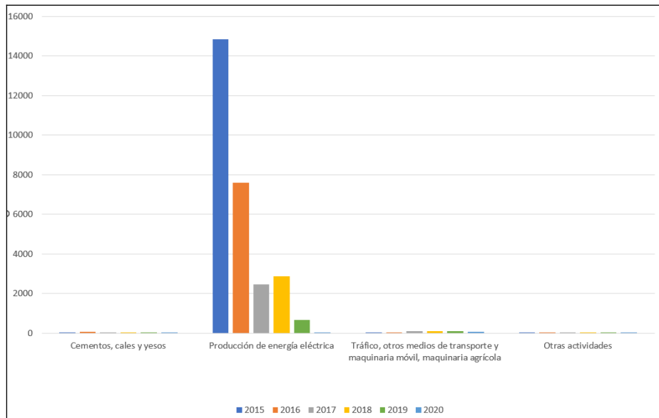
Figura 6.31. Evolución de las emisiones inventariadas de SO 2 (t/año)
