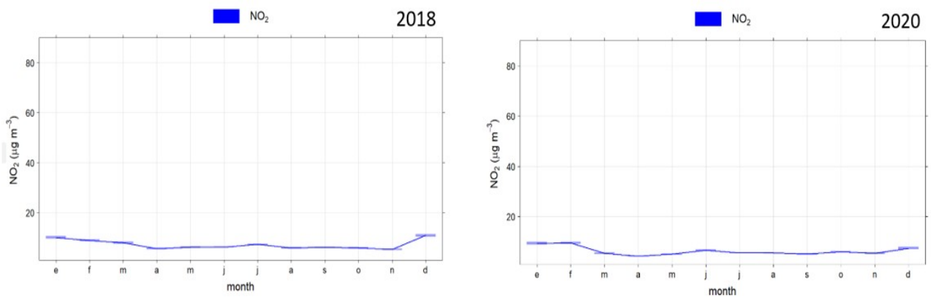
Figura 6.5. Medias mensuales de NO 2 en los años 2018 y 2020. Estación La Granatilla
