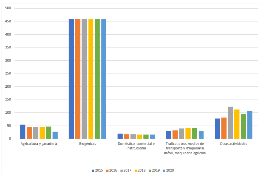
Figura 6.29. Evolución de las emisiones inventariadas de COVNM (t/año)
