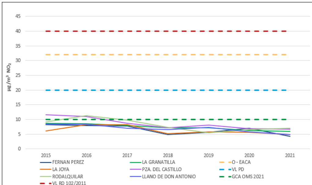
Figura 5.9. Promedio anual de NO 2 (µg/m 3 ) en Zona Industrial de Carboneras
