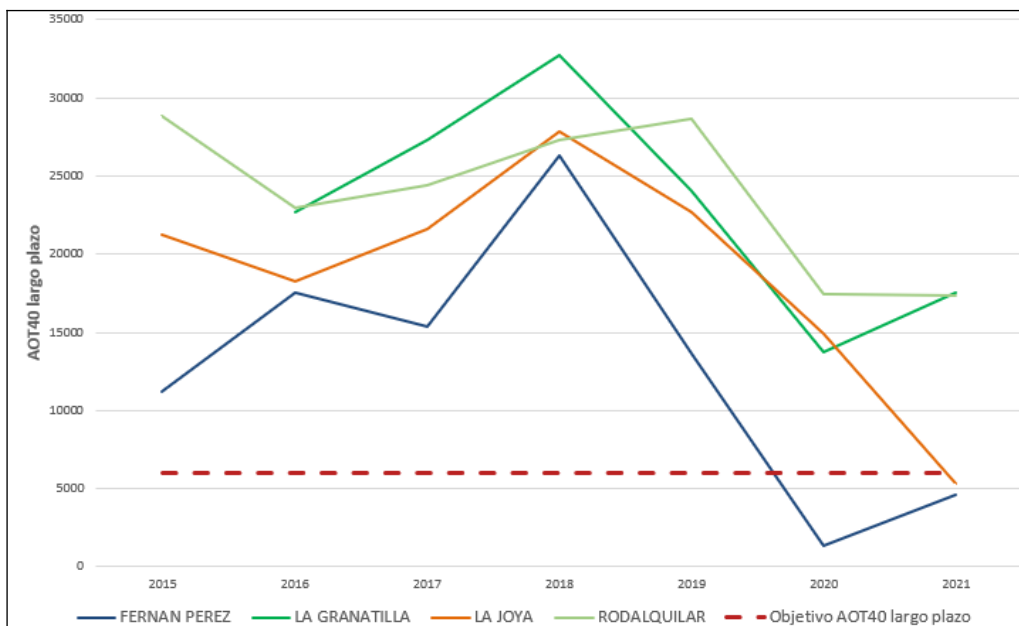
Figura 5.12. AOT40 ( \mu\text{g}/\text{m}^3 \cdot \text{h} ) a largo plazo para Zona Industrial de Carboneras
