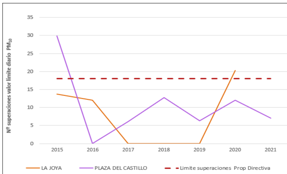
Figura 5.5. Número de superaciones del futuro valor límite diario de PM 10 (propuesta de directiva de calidad del aire) en Zona Industrial de Carboneras
