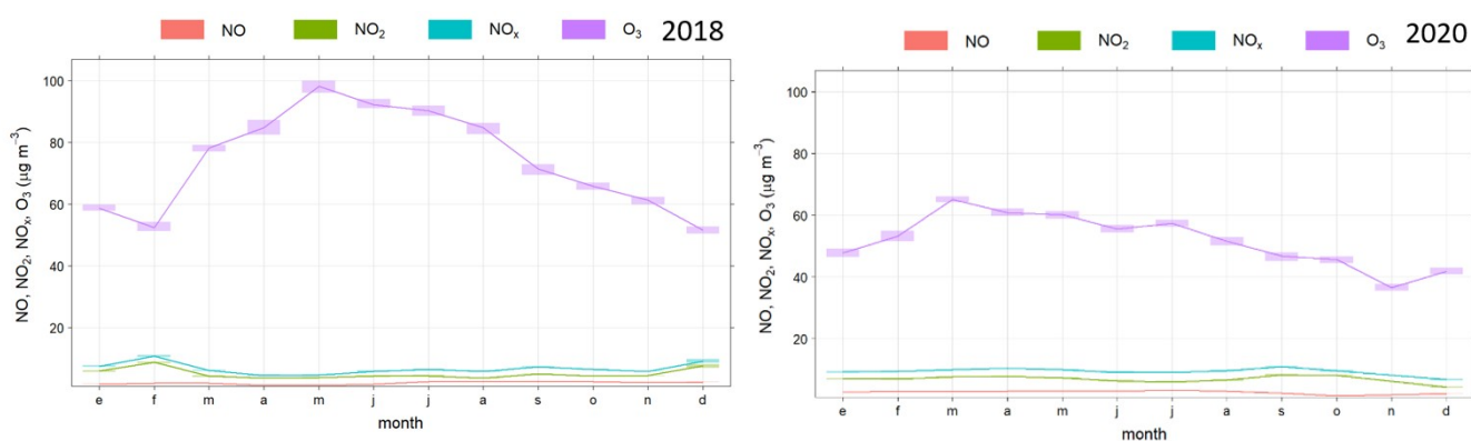
Figura 6.13. Medias mensuales de \text{O}_3 , \text{NO}_x , \text{NO}_2 y \text{NO} en los años 2018 y 2020. Estación Fernán Pérez
