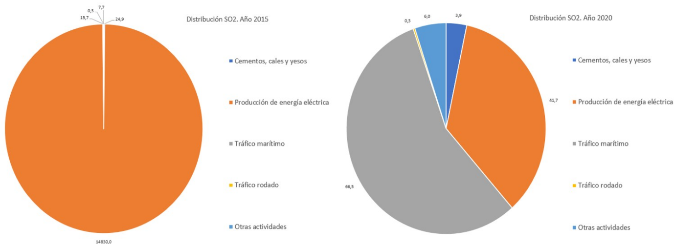
Figura 6.35. Distribución por sectores de las emisiones inventariadas en los años 2015 y 2020 de SO 2 (t/año)
