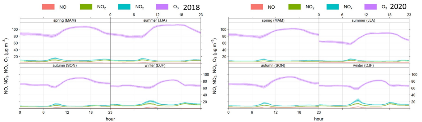
Figura 6.18. Patrón horario estacional para O 3 , NO x , NO 2 y NO en 2018 y 2020. Estación La Granatilla
