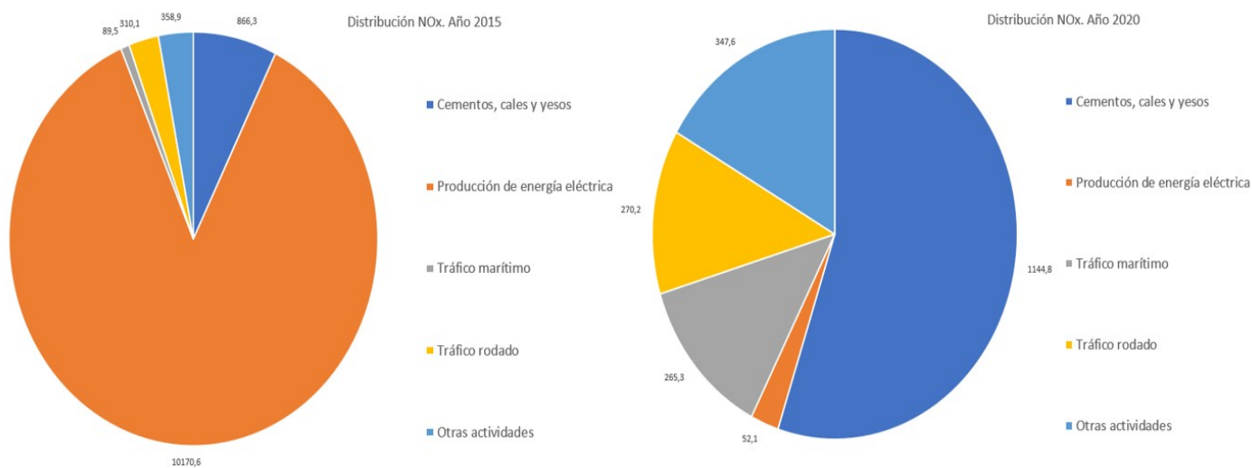
Figura 6.34. Distribución por sectores de las emisiones inventariadas en los años 2015 y 2020 de NO x (t/año)
