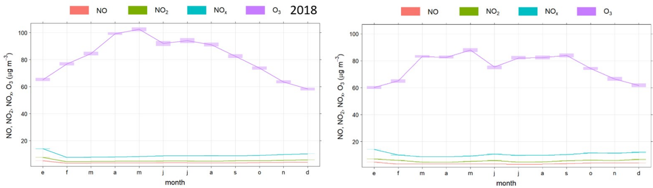
Figura 6.15. Medias mensuales de O 3 , NO x , NO 2 y NO en los años 2018 y 2020. Estación La Joya
