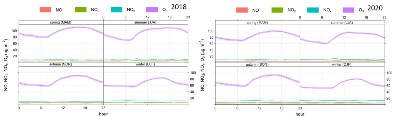
Figura 6.19. Patrón horario estacional para O 3 , NO x , NO 2 y NO en 2018 y 2020. Estación La Joya
