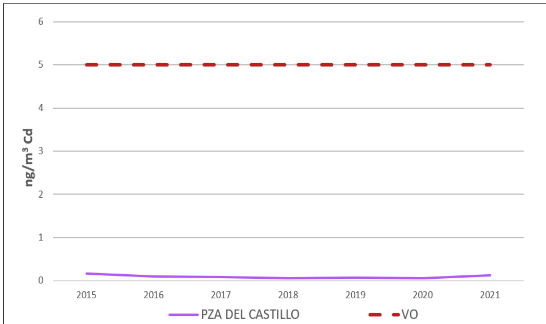
Figura 5.17. Medias anuales de Cd (ng/m³) en Zona Industrial de Carboneras
