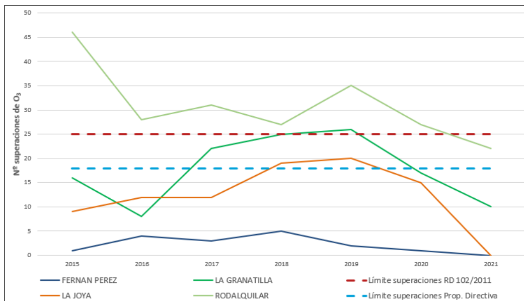
Figura 5.10. Número de superaciones del valor objetivo de ozono para la protección de la salud humana en Zona Industrial de Carboneras
