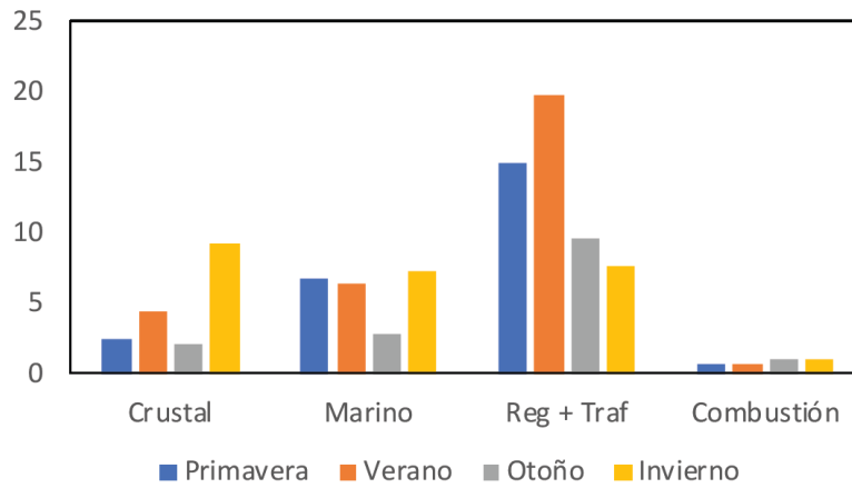
Figura 6.26. Contribución de fuentes por estaciones durante el año 2021 para PM 10 en la estación de Plaza del Castillo
