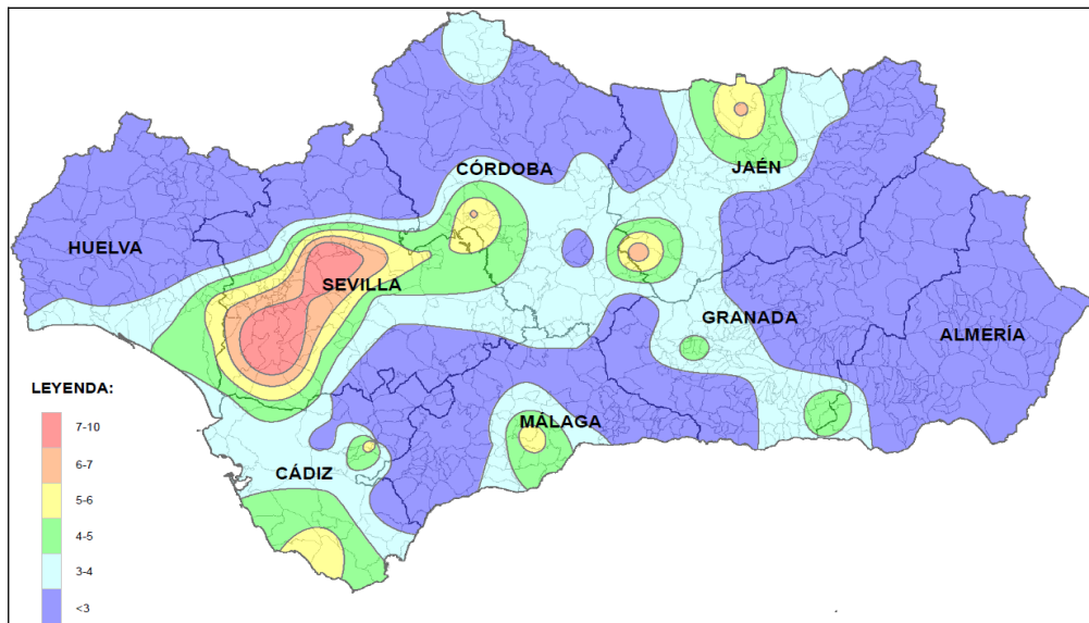
Figura 5.20. Resultados de la campaña de captadores difusivos en fondo rural. Promedio de NO 2 en 2020
