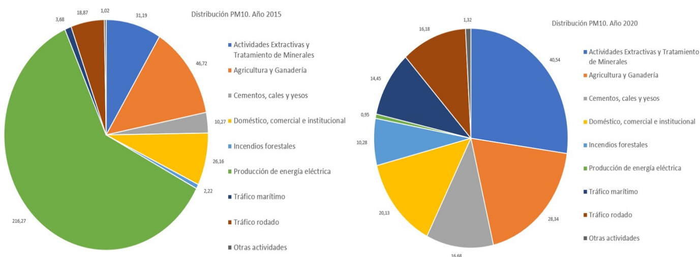
Figura 6.32. Distribución por sectores de las emisiones inventariadas en los años 2015 y 2020 de PM 10 (t/año)
