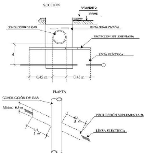
Figura 31: Detalles de cruzamiento y conducciones (ITC-LAT 06).
