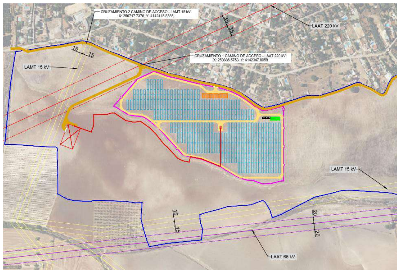
Figura 14: Líneas eléctricas existentes.
