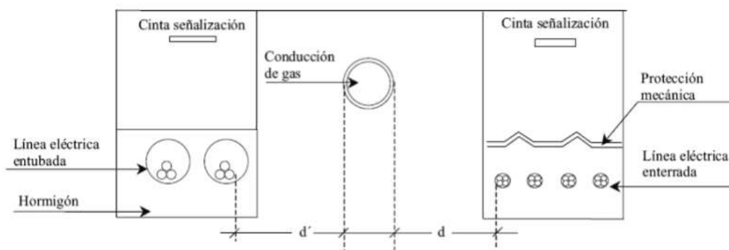
Figura 33: Detalles de paralelismo y conducciones (ITC-LAT 06).
