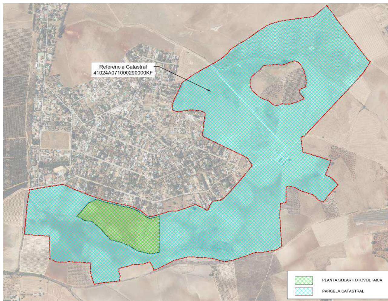
Figura 2 .Área disponible para la Implantación de la Planta Solar FV
