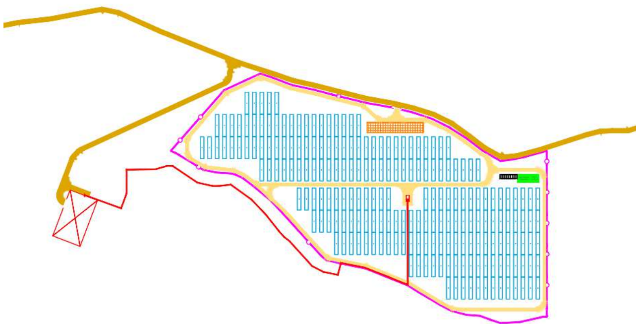
Figura 23: Planta Solar FV.
