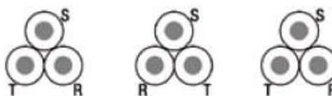
Figura 28: Colocación de cables en tresbolillo.
