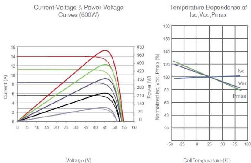
Figura 25: Curvas Características JKM600N-78HL4.
