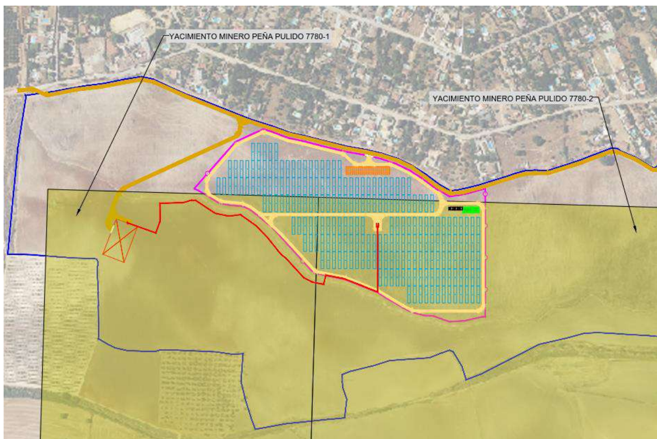
Figura 21. Yacimientos mineros Zona de Estudio
