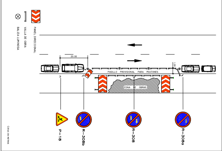
SEÑALIZACIÓN DE OBRAS EN LA VÍA PÚBLICA (Ocupación total de la obra "A")
