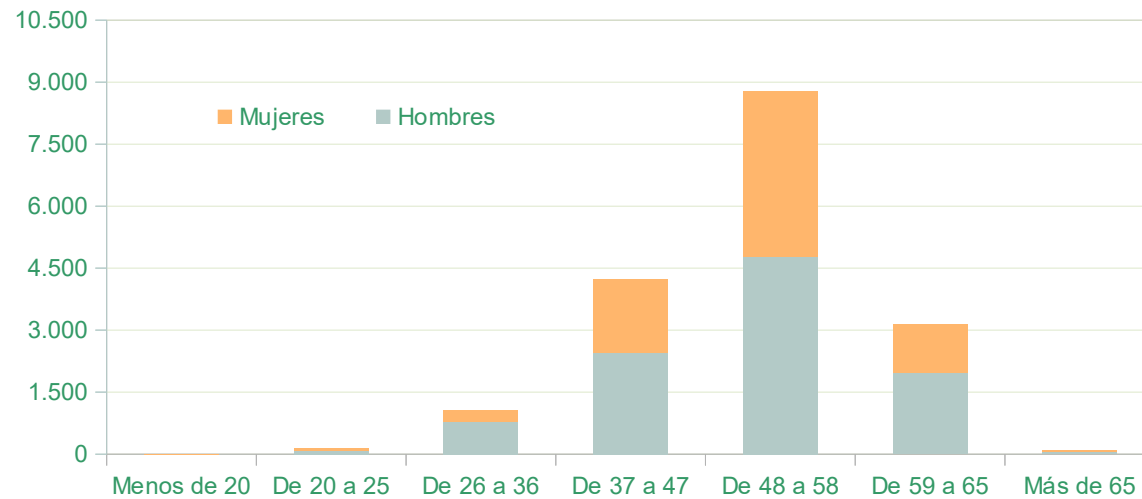
Distribución del número de efectivos a 31 de diciembre de 2024 según grupo de edad y sexo
