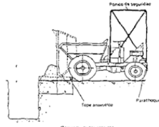
Carretilla autovoltante
