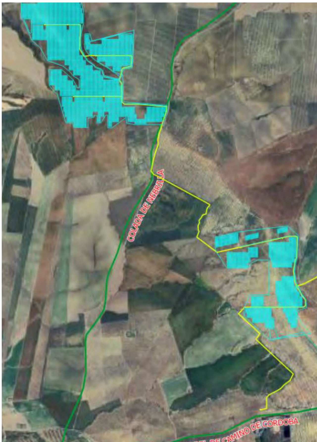
Planta Solar Fotovoltaica Alcudia Solar, línea de evacuación en media tensión y vía pecuaria (“COLADA DE NEBRILLA”) en el entorno del proyecto coincidente con el Camino de Morente.
