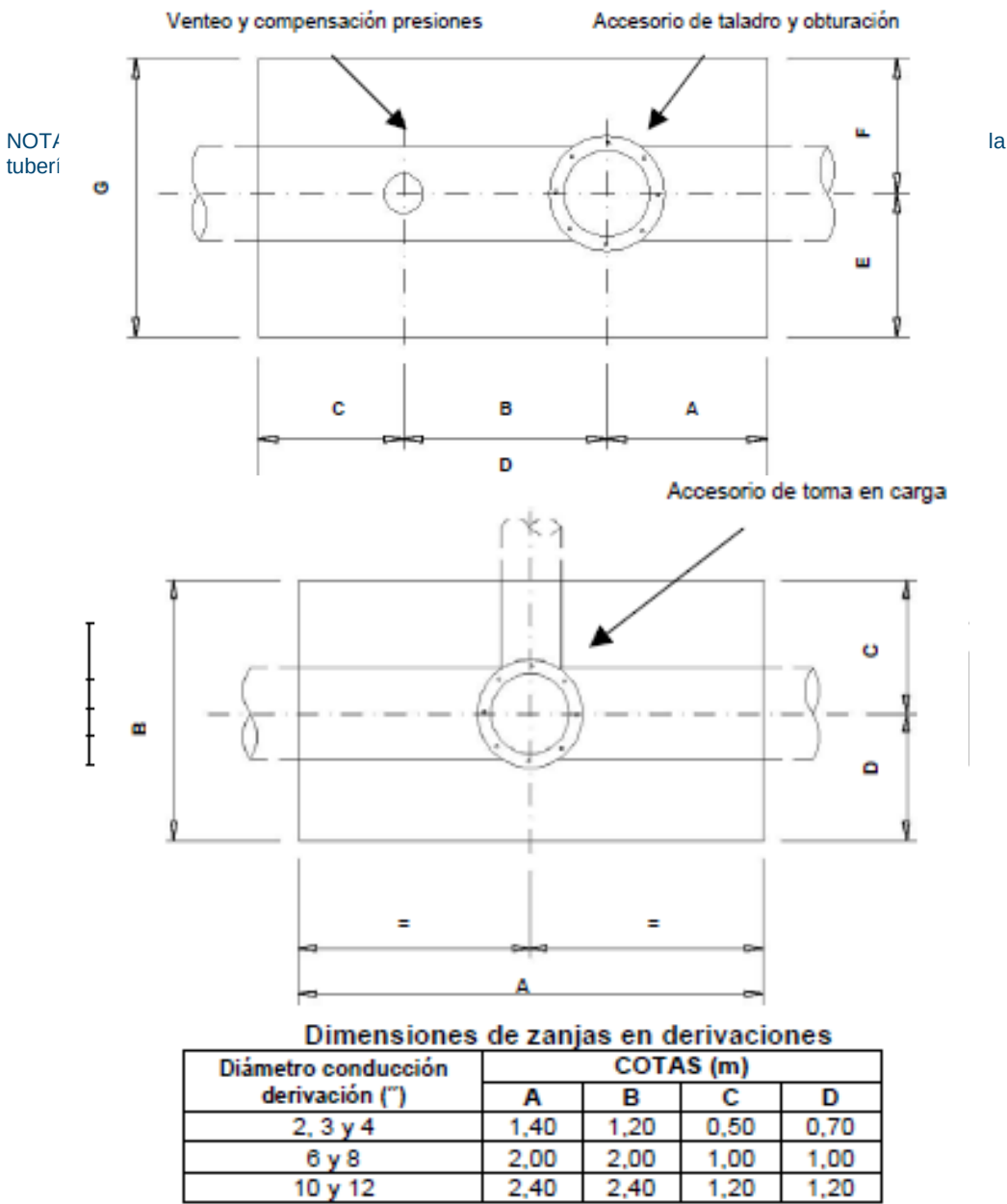
Figura.1-Dimensiones de zanjas en Taladros Simples
