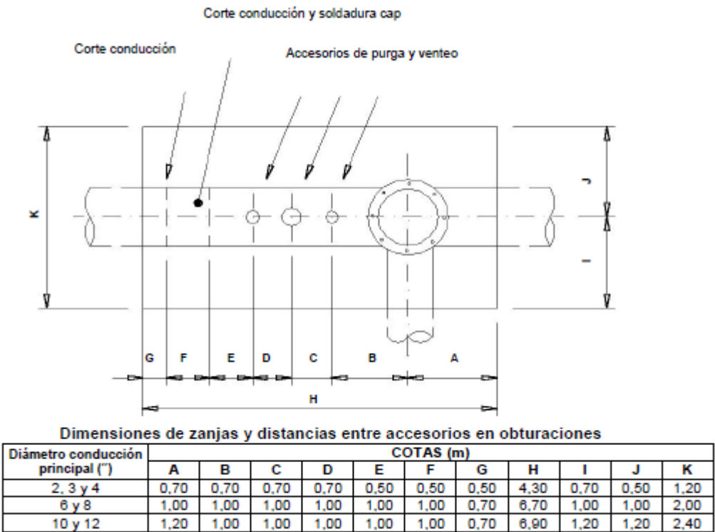
Figura.3-Dimensiones de zanjas y distancia entre accesorios en obturaciones
