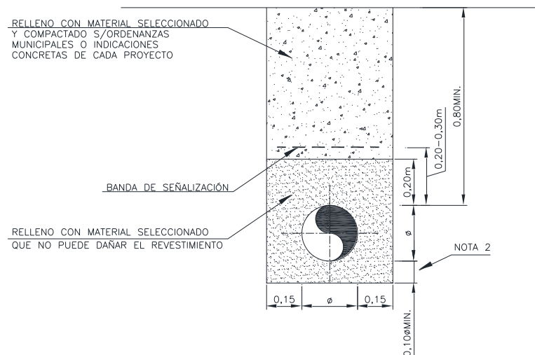
b) Perfil de coronación llano
