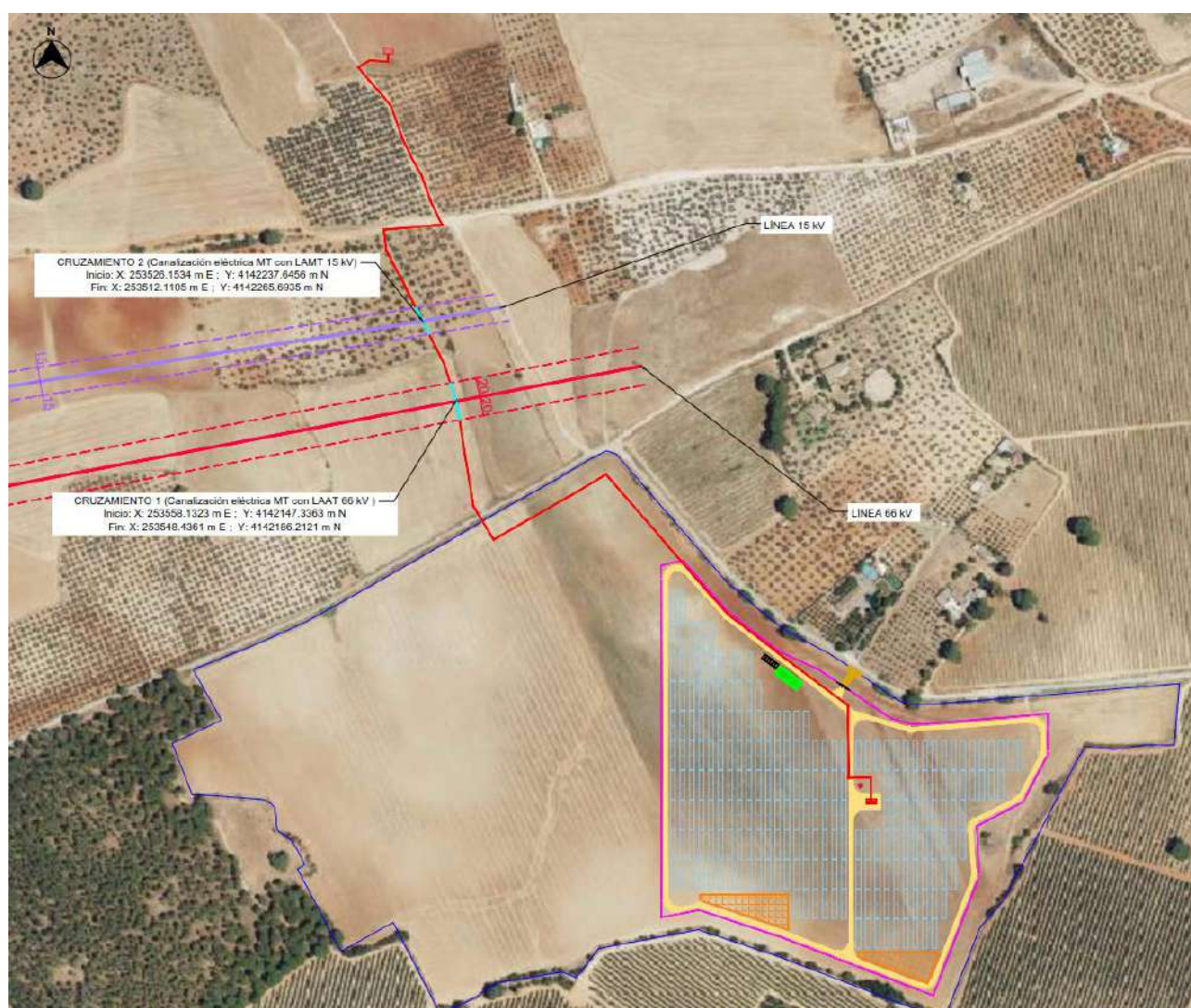
Figura 12. Líneas eléctricas existentes.
