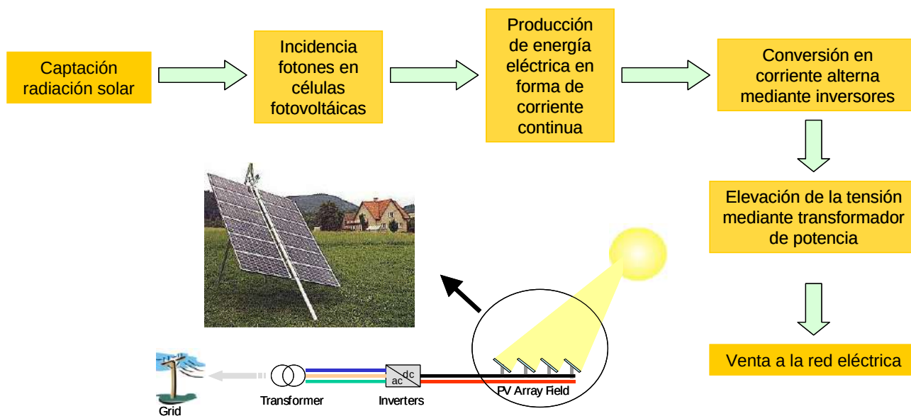
Figura 18: Principio de Funcionamiento Instalación FV.
