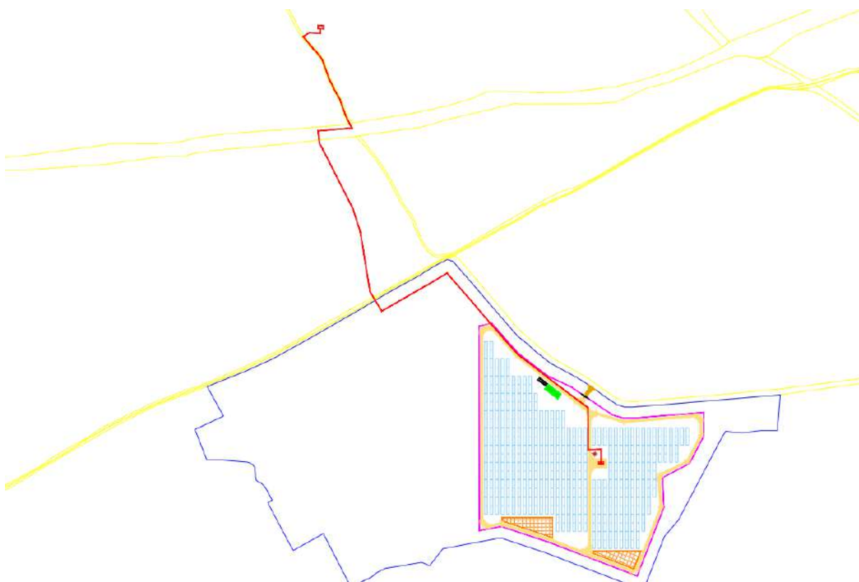
Figura 19: Instalación FV.
