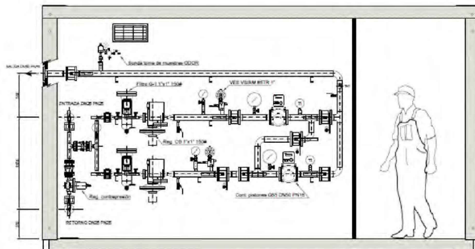
SECCION A-B
