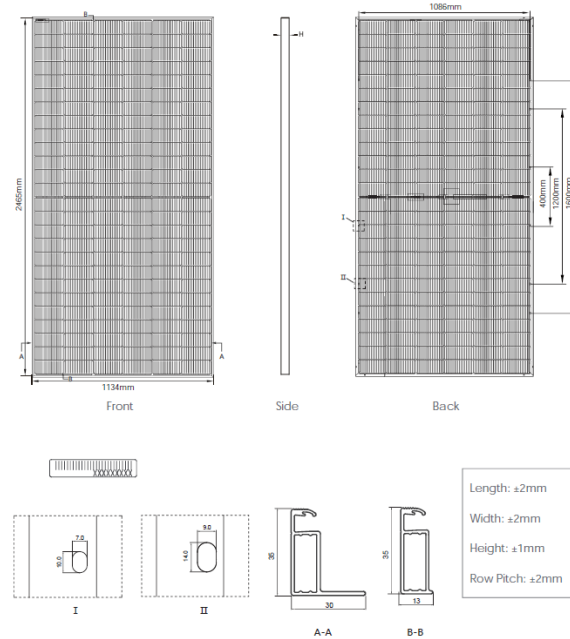
Figura 20: Dimensiones del Módulo.
