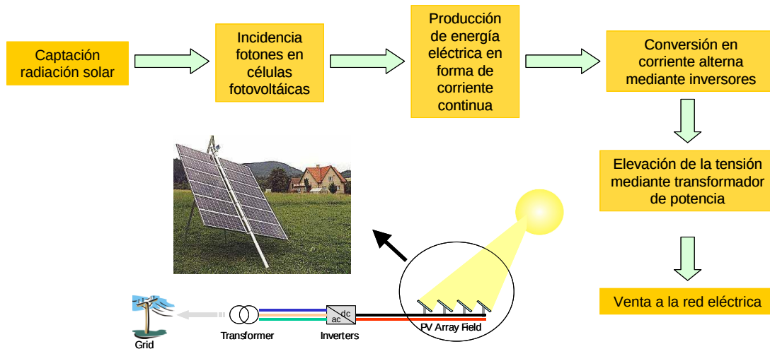
Figura 18: Principio de Funcionamiento Instalación FV.
