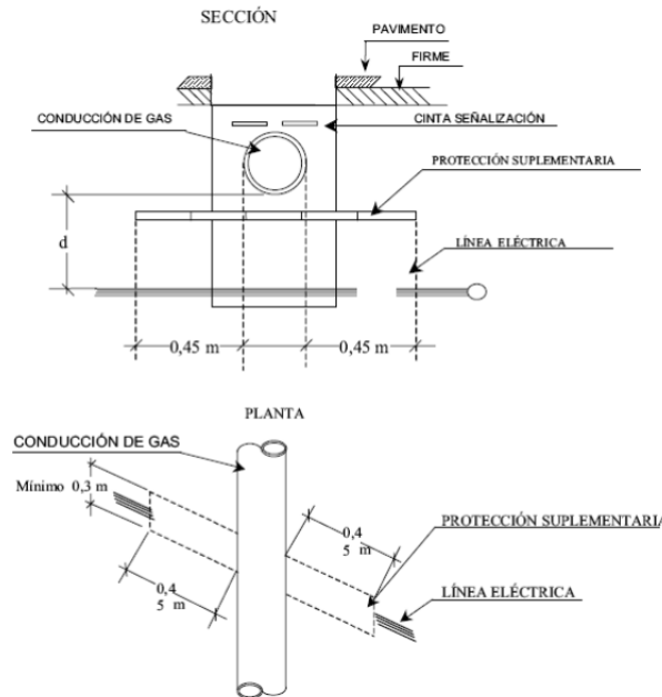
Figura 27: Detalles de cruzamiento y conducciones (ITC-LAT 06).
