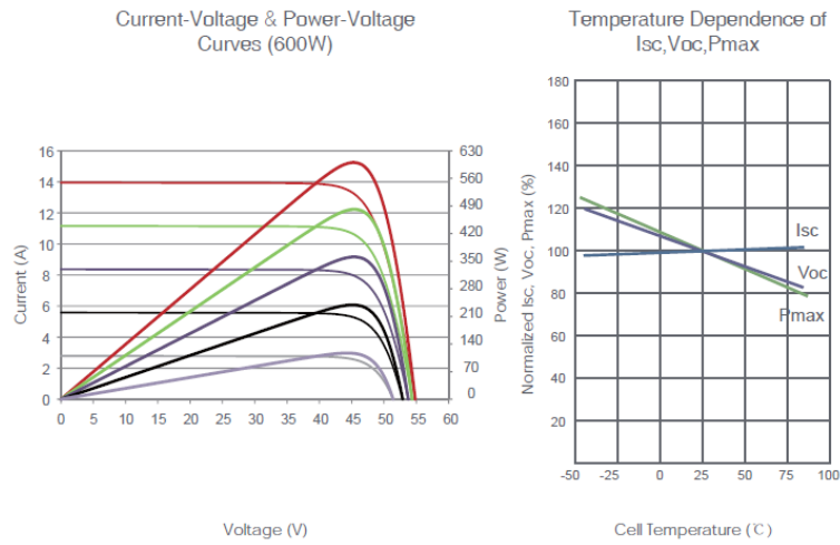
Figura 21: Curvas Características JKM600M-78HL4.
