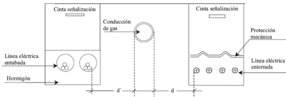
Figura 29: Detalles de paralelismo y conducciones (ITC-LAT 06).
