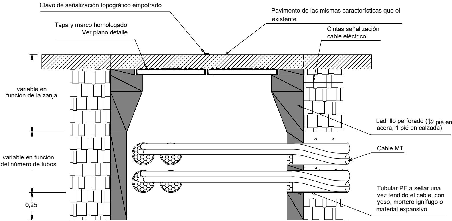
SECCIÓN A-A'
