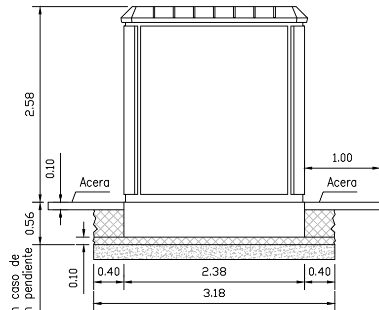
VISTA LATERAL
