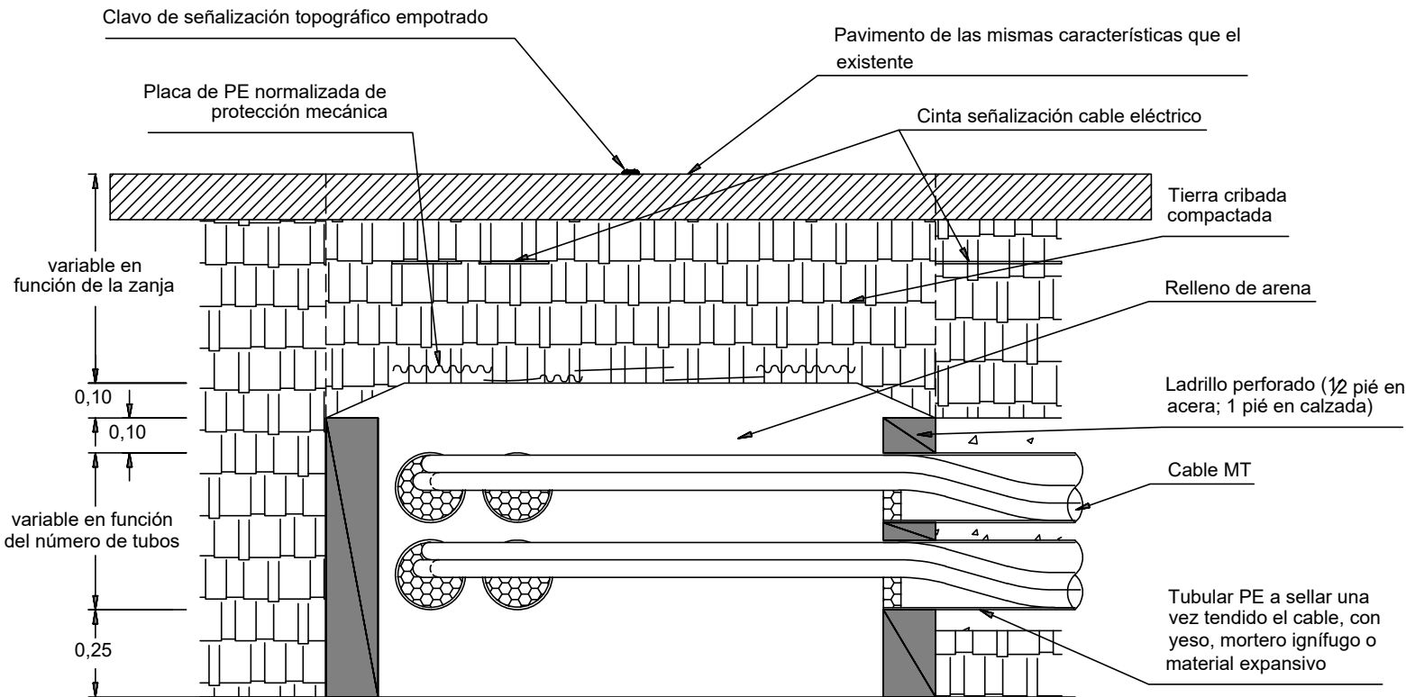
SECCIÓN A-A'
