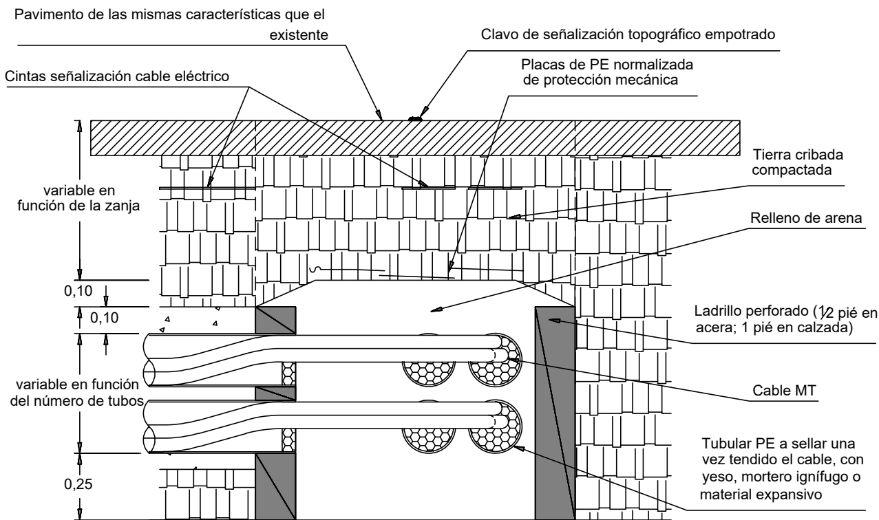
SECCIÓN B-B'
