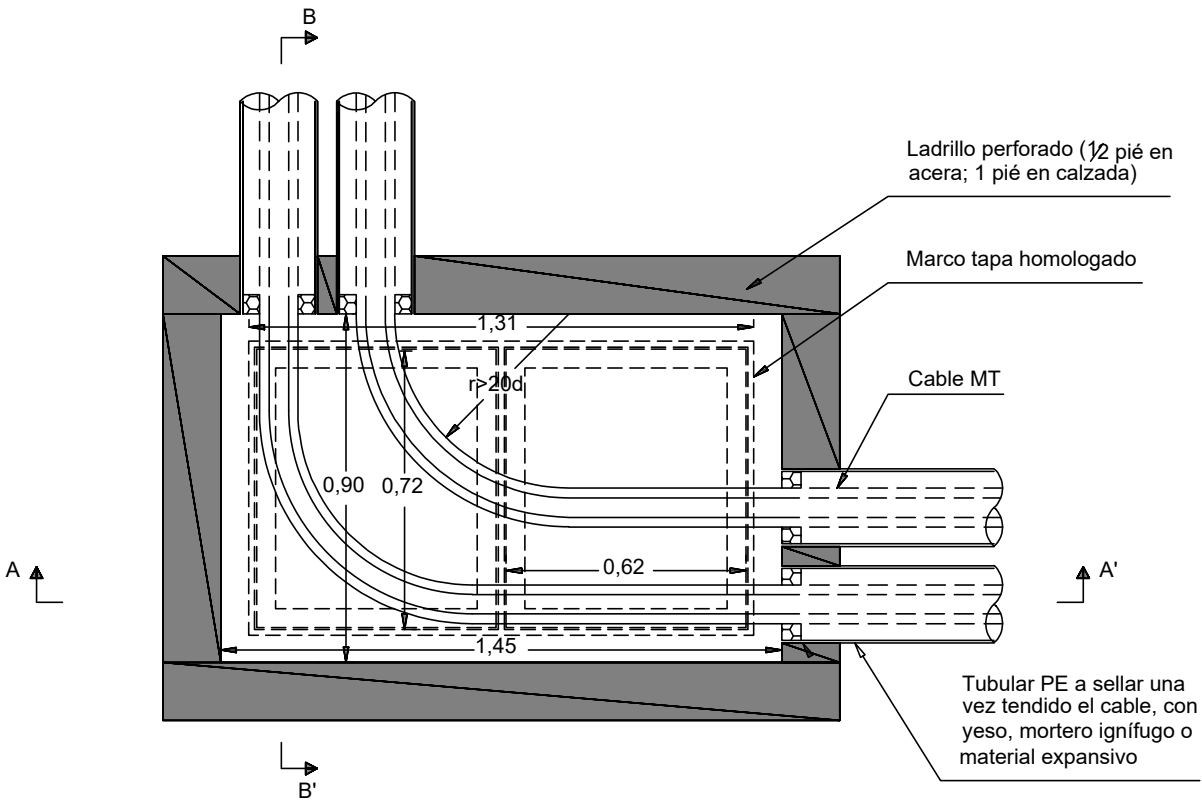
PLANTA
