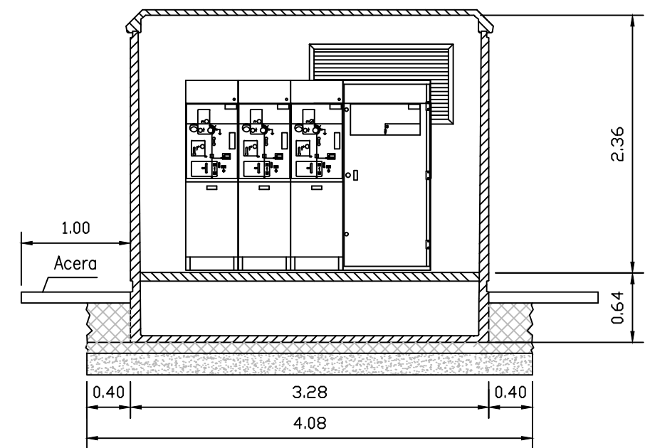
SECCIÓN A-A
