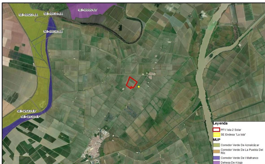
Figura 97. Montes de Utilidad Pública. Fuente WMS Catalogo de Montes públicos de Andalucía.
