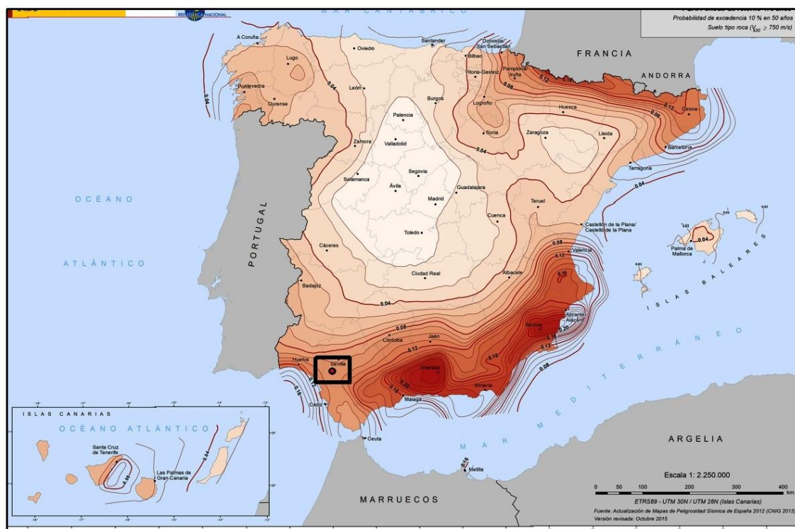
Figura 127. Mapa de peligrosidad sísmica en términos de aceleración. Fuente: IGN
