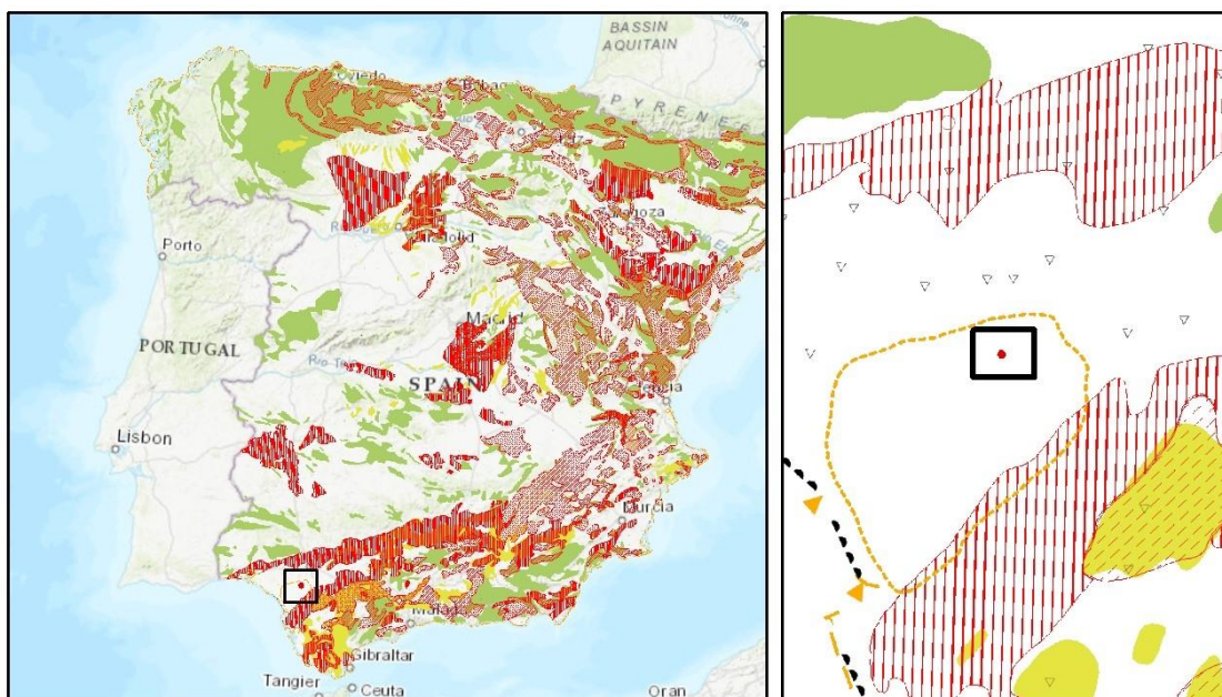
Figura 128. Mapa de Movimientos del Terreno de España escala. Fuente: IGME
