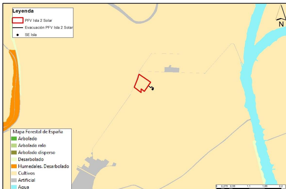
Figura 74. Vegetación y usos de suelo. Fuente: Mapa Forestal de España, 2018.
