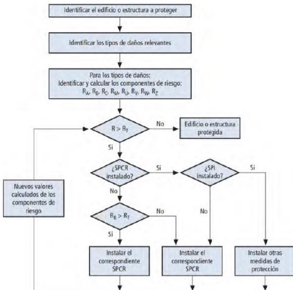
Ilustración 18. Diagrama de flujo para la elección de medidas de protección para los tipos de pérdida
