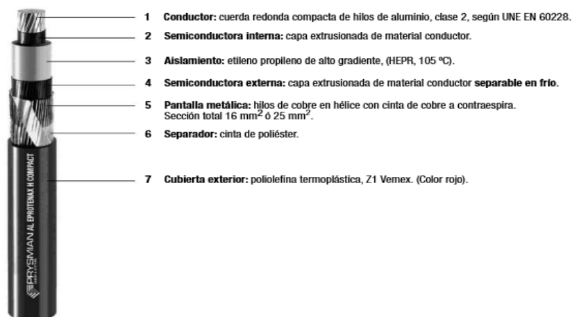
Ilustración 21. Componentes del conductor de Aluminio (Al)
