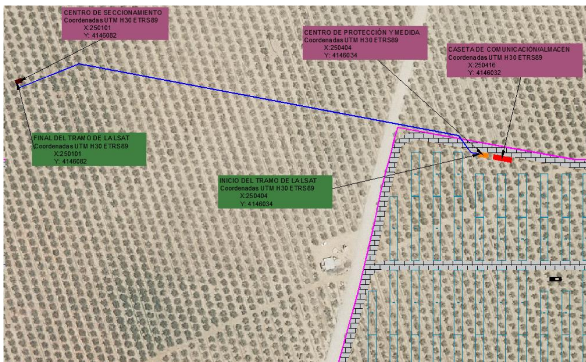
Ilustración 31. Situación del tramo subterráneo (Fuente: Propia)
