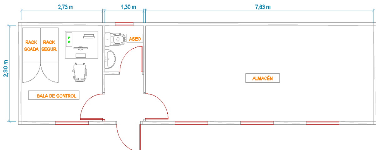
Ilustración 11. Imagen del edificio
