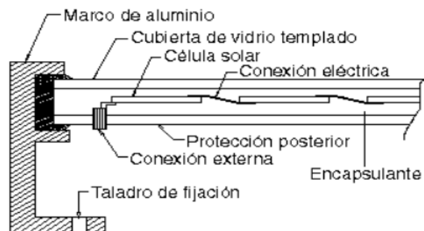
Ilustración 12. Representación del corte longitudinal de un módulo fotovoltaico (Fuente: Externa)
