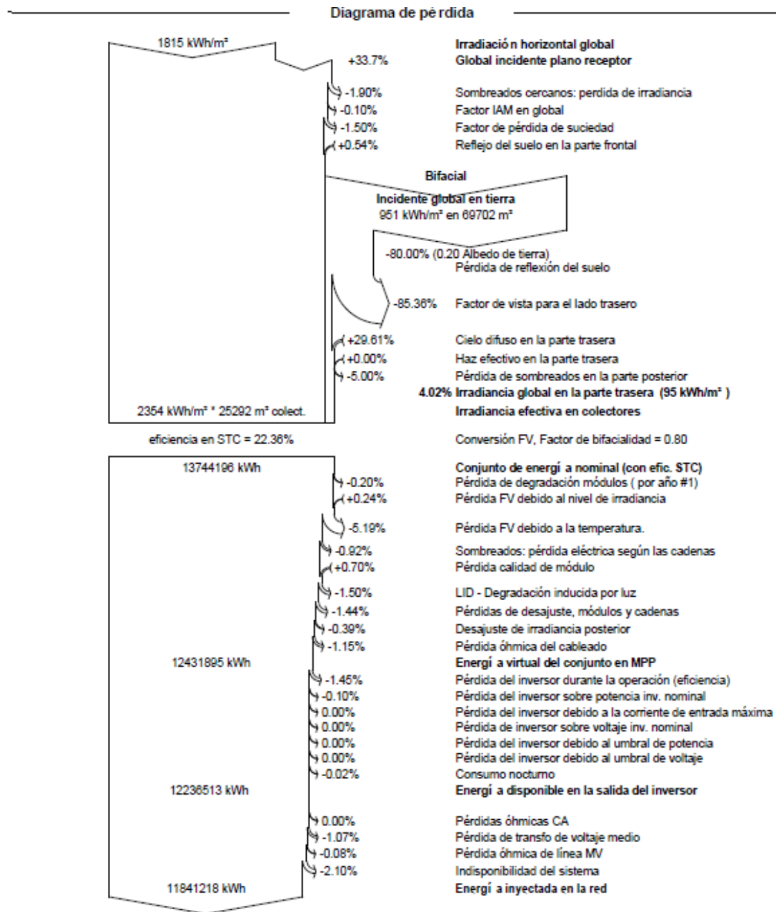
Ilustración 17. Desglose de la pérdidas estimadas
