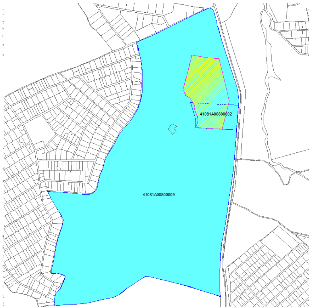
Ilustración 4. Parcelario de la planta solar “Aljarafe 8”
