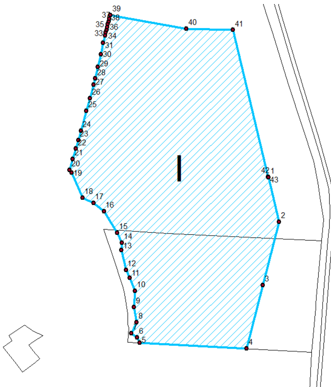
Ilustración 3. Islas de la instalación y puntos del vallado(Fuente: Propia)
