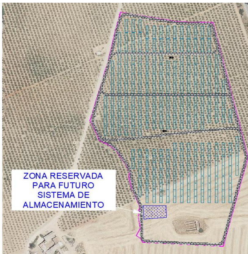
Ilustración 14. Ubicación del futuro sistema de baterías (Fuente: Propia)
