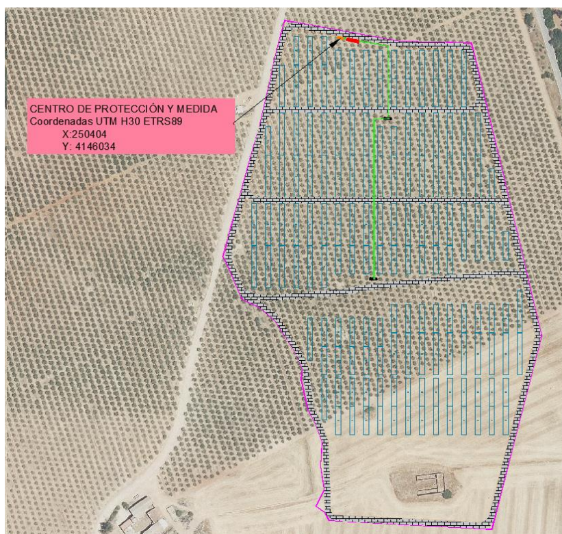
Ilustración 24. Ubicación del CPyM
