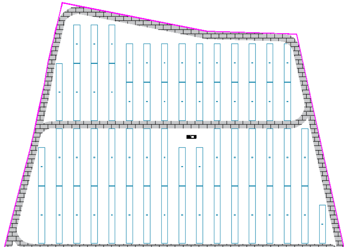
Ilustración 16. Disposición de los módulos alineados (Fuente: Propia)
