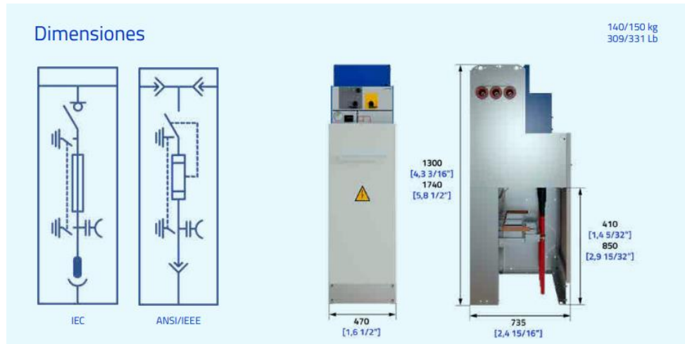
Ilustración 28. Celda modular con protección con fusibles- cgmcosmos-p
