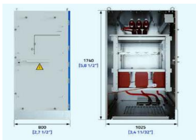
Ilustración 30. Celda modular de medida con aislamiento en aire - cgmcosmos-m
