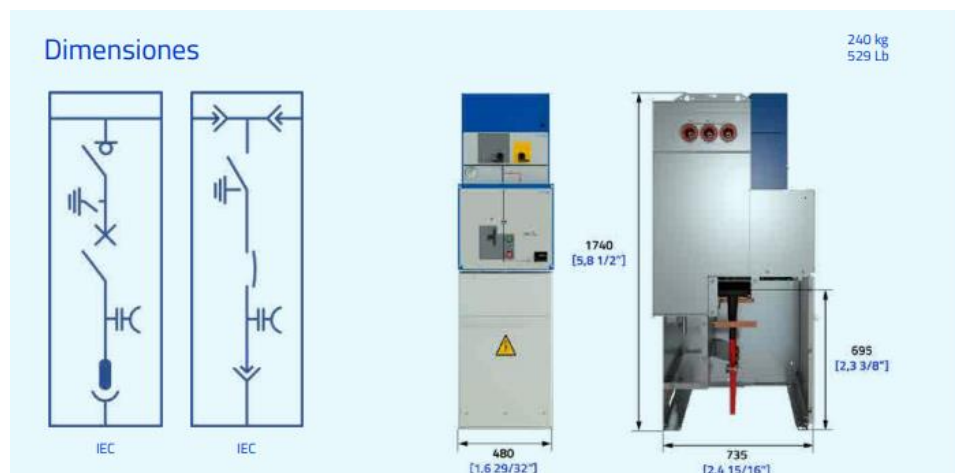
Ilustración 29. Celda modular de protección mediante interruptor automático - cgmcosmos-v
