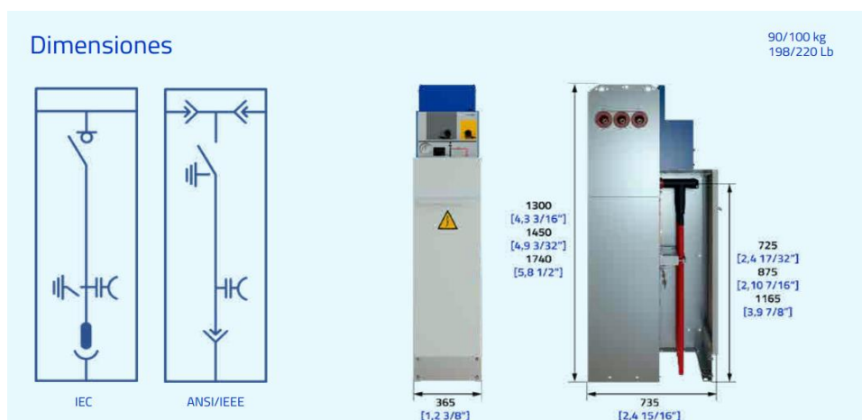
Ilustración 27. Celda modular de línea cgmcosmos-l
