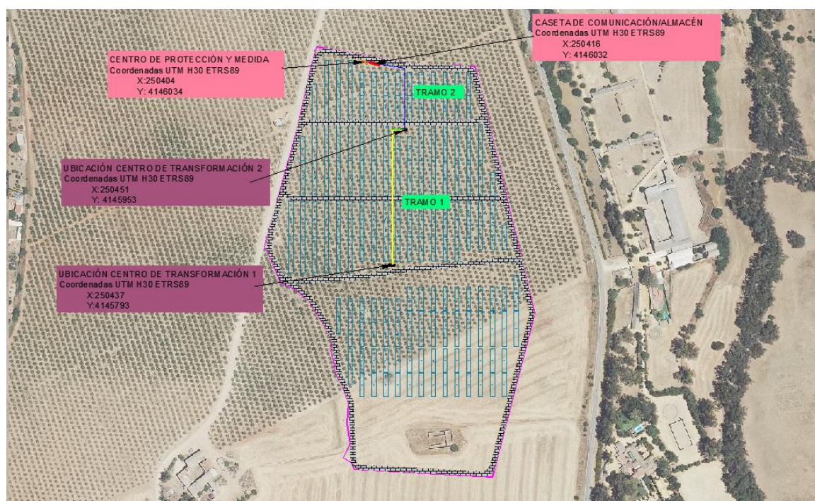
Ilustración 20. Situación del ramal (Fuente: Propia)
