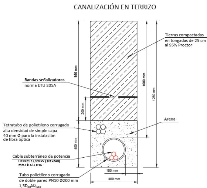
Ilustración 32. Zanjas asociada a una línea subterránea de evacuación
