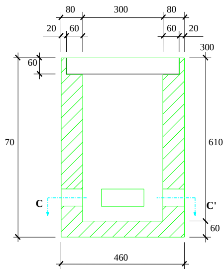
SECCIÓN B-B'
